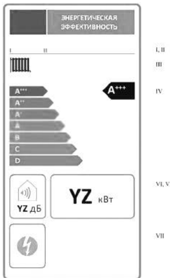
Рисунок Б.2 — Вид этикетки энергетической эффективности устройства для отопления помещений с комбинированной выработкой тепловой и электрической энергии классом сезонной энергетической эффективности от A+++ до D
