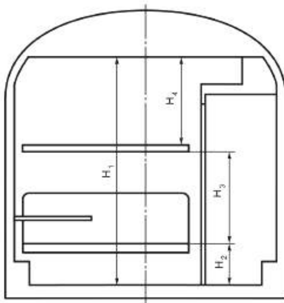
Рисунок 1 — Поперечное сечение купейного вагона
