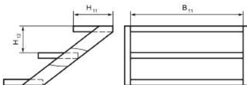
Рисунок 17 — Ступеньки при входе в вагон
