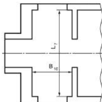
Рисунок 16 — Тамбур
