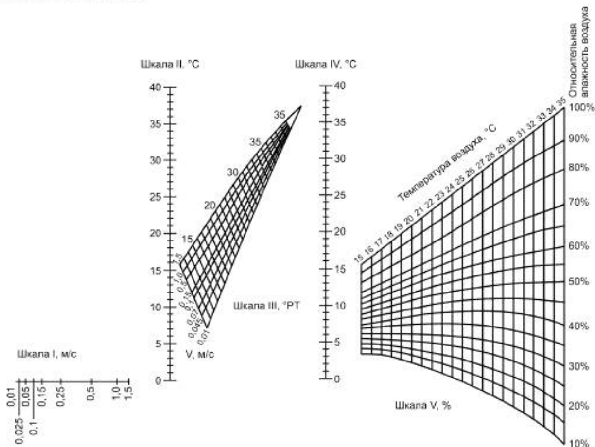
Рисунок В.1 — Номограмма для определения результирующей температуры ( t_{PT} ) по установленным параметрам микроклимата в помещениях вагона
