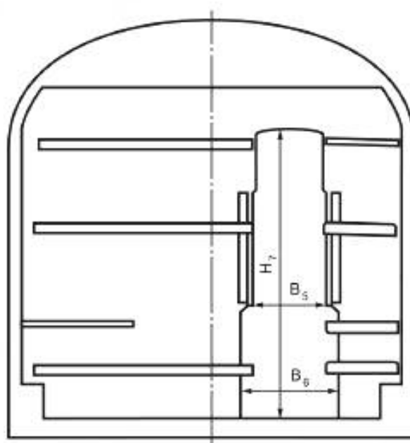
Рисунок 5 — Поперечное сечение вагона открытого типа
