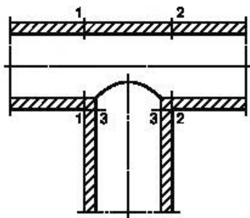
Рисунок 12 — Расчетные сечения тройникового узла
