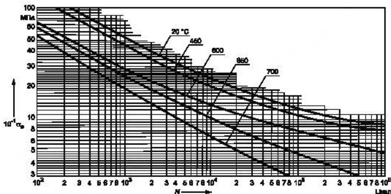
Рисунок 4 — Расчетные кривые малоциклового усталости аустенитных хромоникелевых сталей
