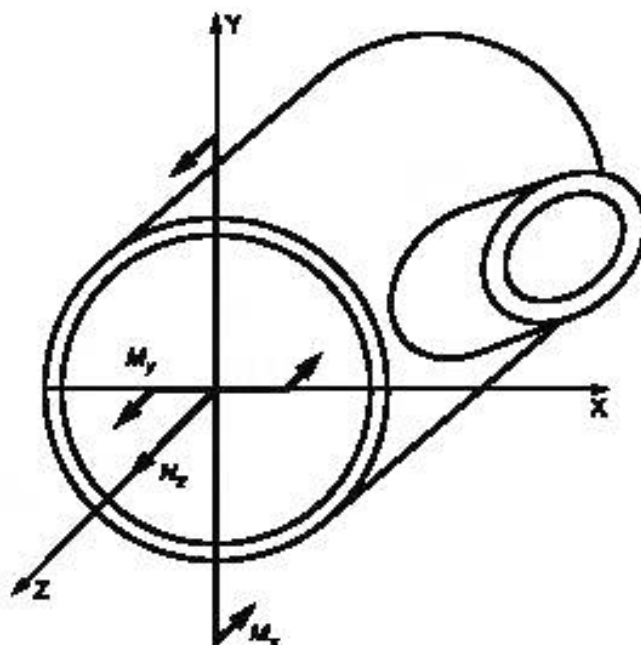
Рисунок 14 — Силовые факторы в поперечном сечении тройникового узла
