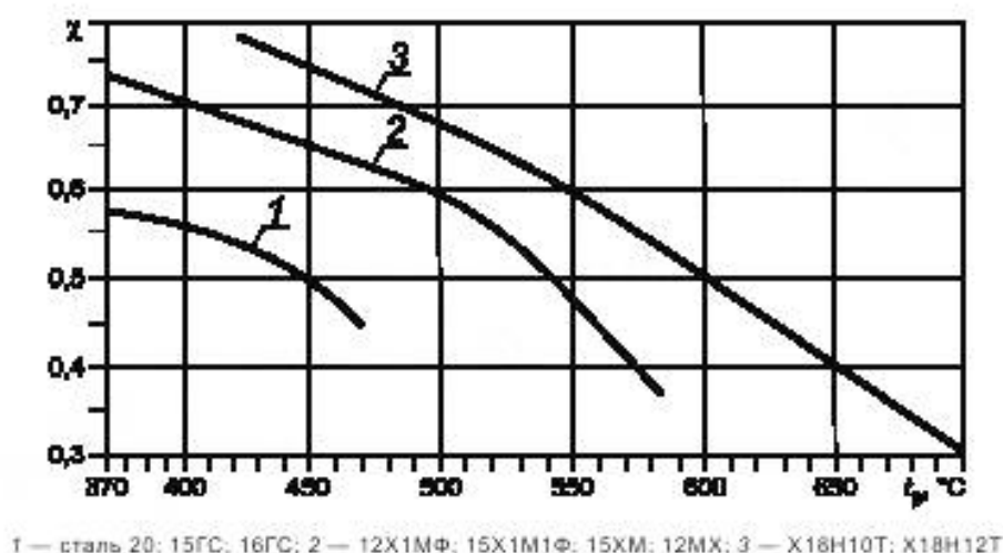
Рисунок 5 — Коэффициент усреднения компенсационных напряжений
