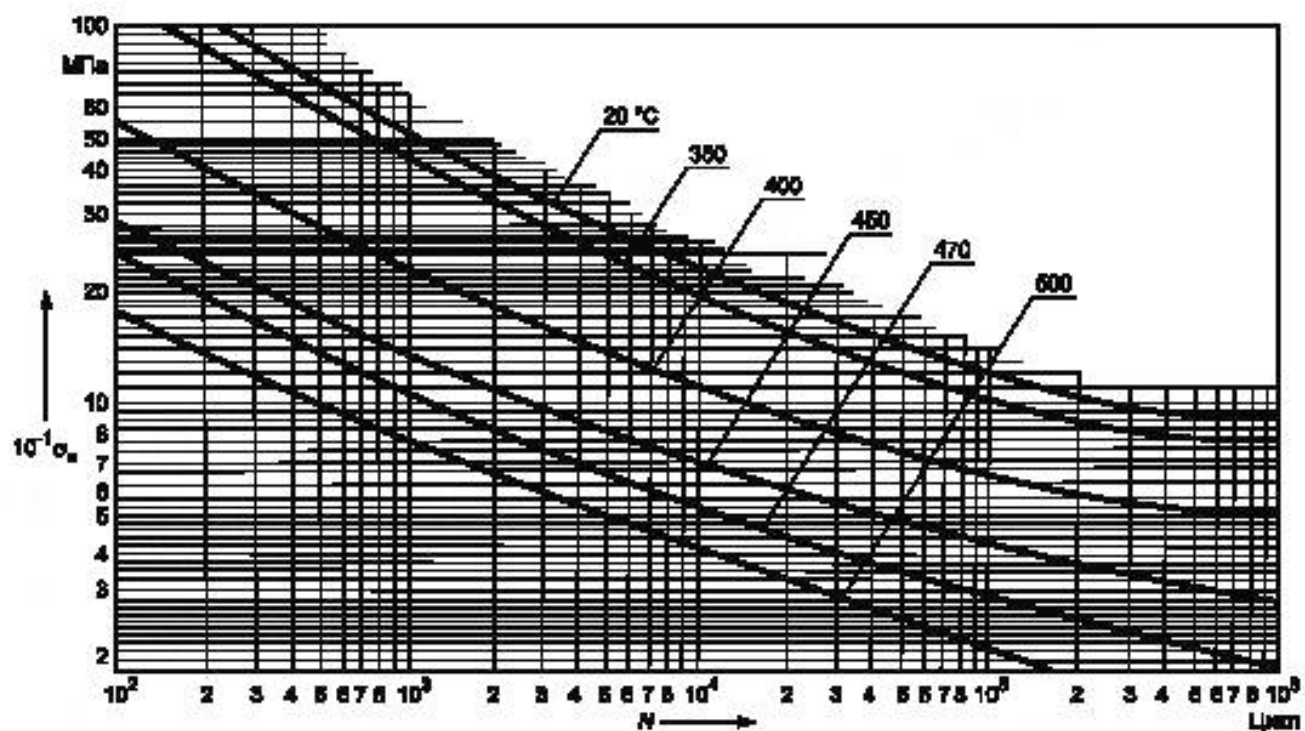
Рисунок 2 — Расчетные кривые малоциклового усталости углеродистых сталей
