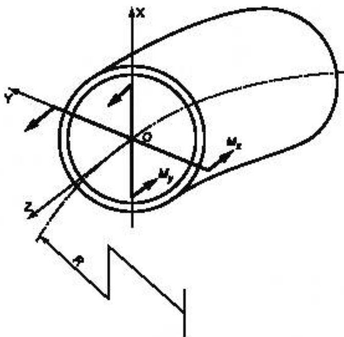
Рисунок 13 — Изгибающие моменты в сечении криволинейной трубы
