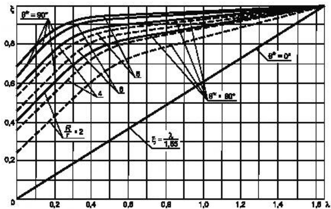
Рисунок 8 — Коэффициент \xi
