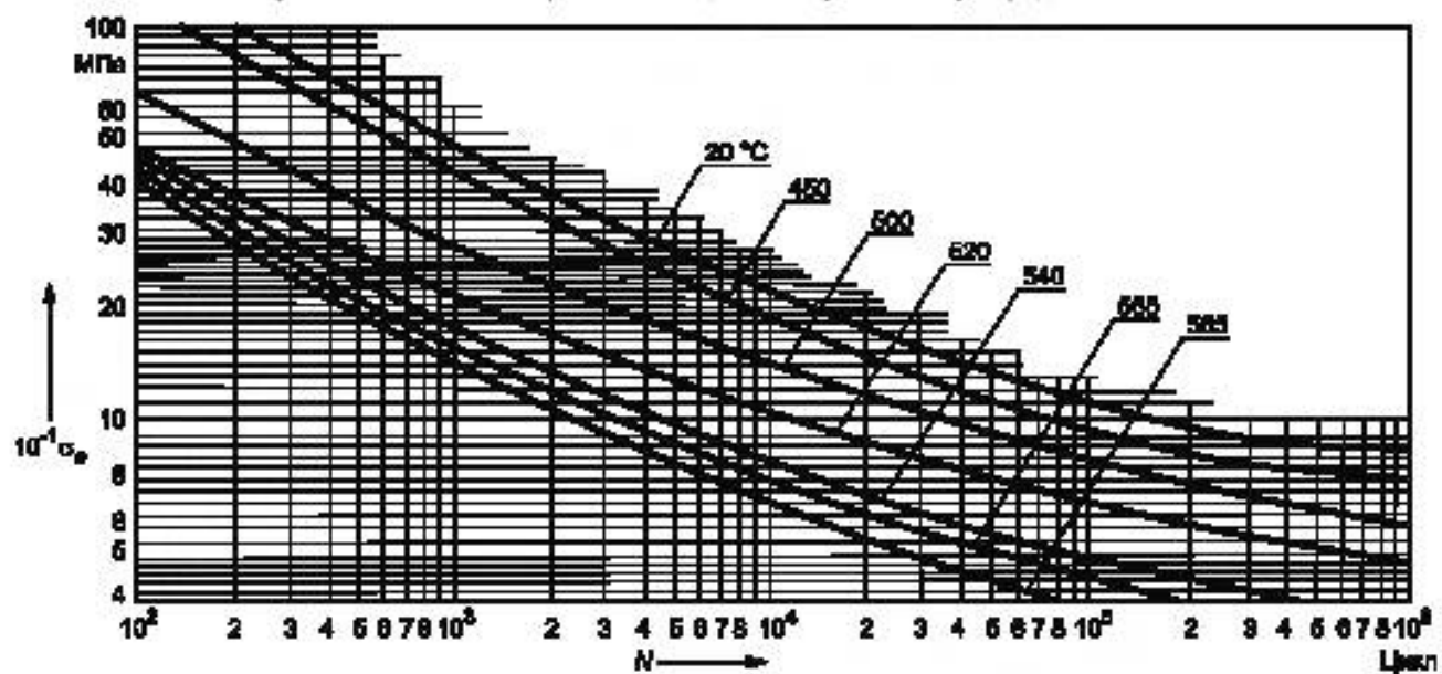
Рисунок 3 — Расчетные кривые малоциклового усталости низколегированных сталей марок 12X1MФ, 15X1M1Ф, 12MX и 15XM
