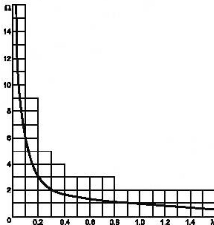
Рисунок 10 — Коэффициент \Omega
