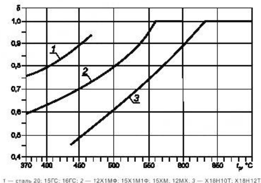
Рисунок 6 — Коэффициент релаксации компенсационных напряжений
