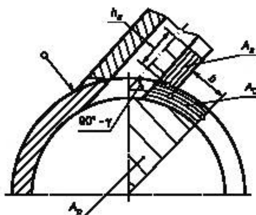
Рисунок 21 — Схема детали с тангенциальным вводом штуцера
