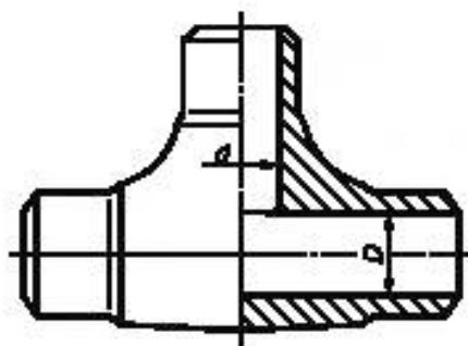
Рисунок 22 — Схема ковкого тройника
