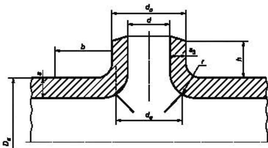
Рисунок 13 — Вытянутая горловина
