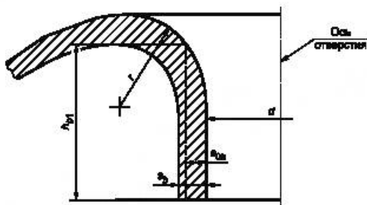
Рисунок 14 — Отбортованный воротник
