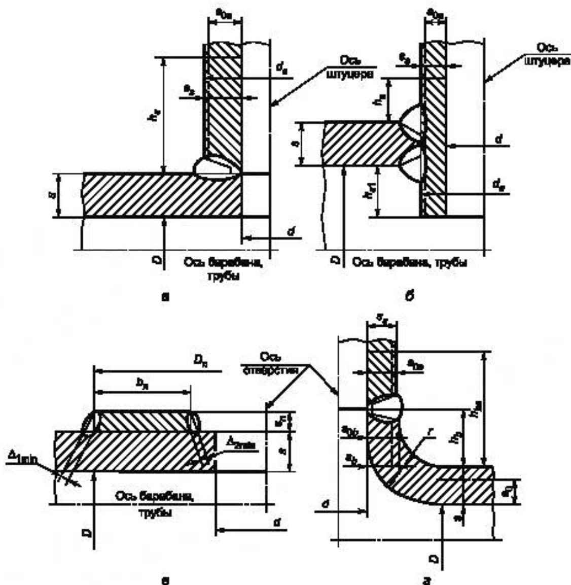
а — укрепление наружным штуцером; б — укрепление проходным штуцером; в — укрепление накладкой; г — укрепление вытянутой горловиной; s_{ob} = s_{os} при одинаковой марке стали
