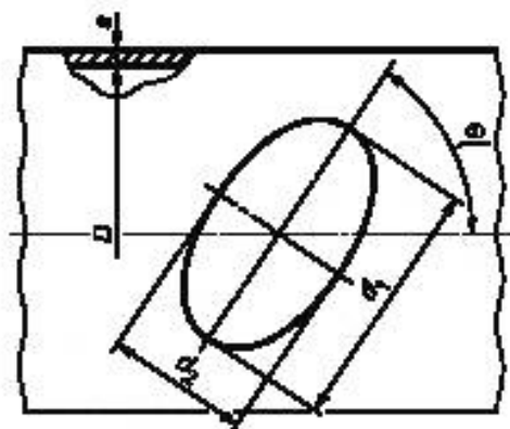
Рисунок 15 — Отверстие эллиптической формы
