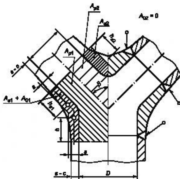
Рисунок 24 — Схема развилки
