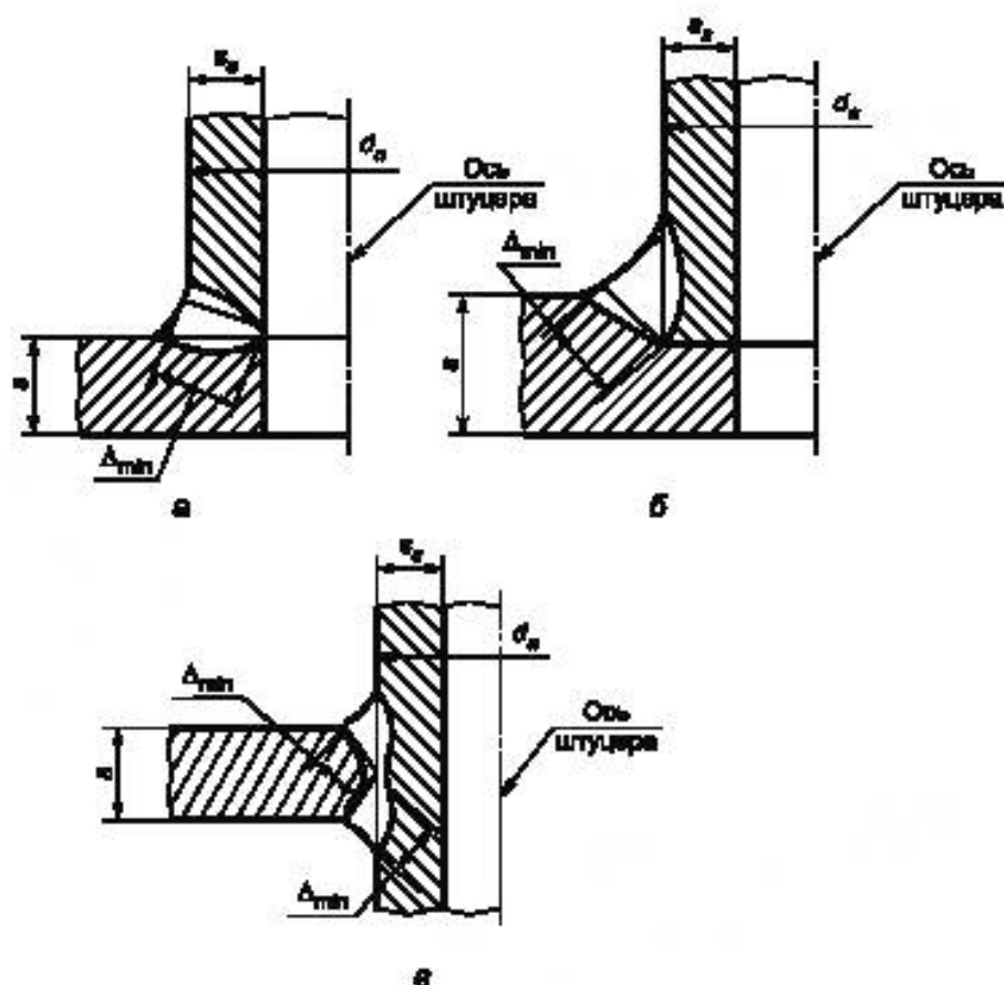
а — шов наружного штуцера; б — шов утопленного штуцера; в — шов проходного штуцера
