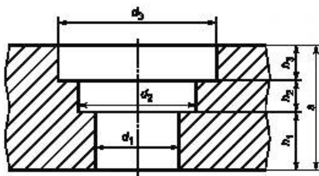
Рисунок 12 — Отверстие с различными диаметрами по толщине стенки
