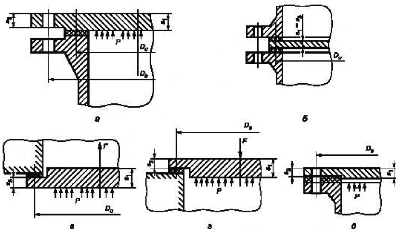
Рисунок 7 — Круглые плоские крышки (заглушки)
