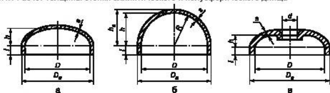
а — глухое эллиптическое днище; б — глухое полусферическое днище; в — эллиптическое днище с лазовым отверстием
