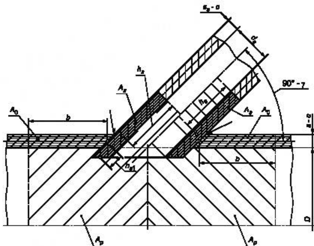
Рисунок 20 — Схема детали с наклонным штуцером
