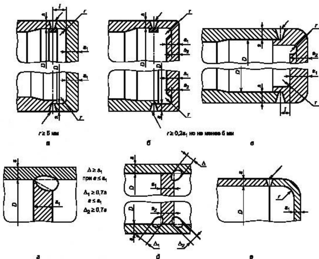
Рисунок 4 — Типы плоских донц
