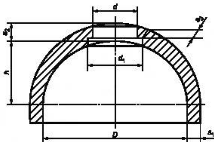
Рисунок 3 — Лазерное отверстие в выпуклом днище переменной толщины
