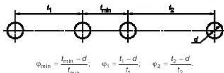
Рисунок 16 — Ряд из четырех отверстий с неравномерным шагом
