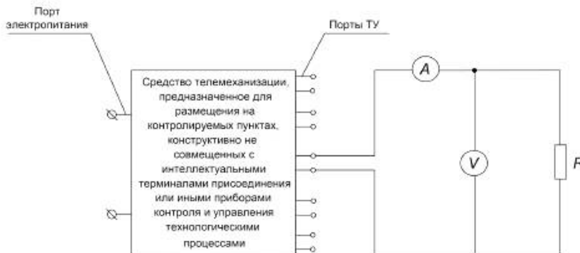
Рисунок 2 — Схема проверки параметров сигнала ТУ
