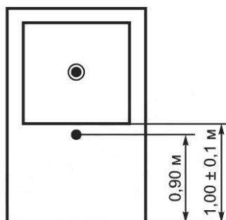
д – створка двери со стеклянной панелью на высоте более 1,0 м
