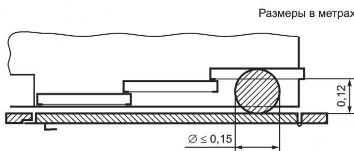
Рисунок 9 — Распашная дверь шахты и горизонтально-раздвижная дверь кабины
