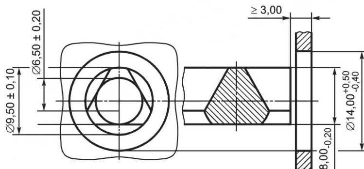
Рисунок 13 — Ключевина
