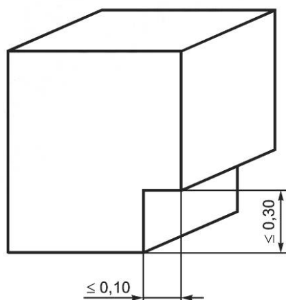
Рисунок 4 — Максимальные уменьшения пространств безопасности для персонала
