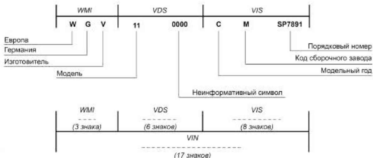
Рисунок Б.3 — Пример № 3 построения кода VIN
