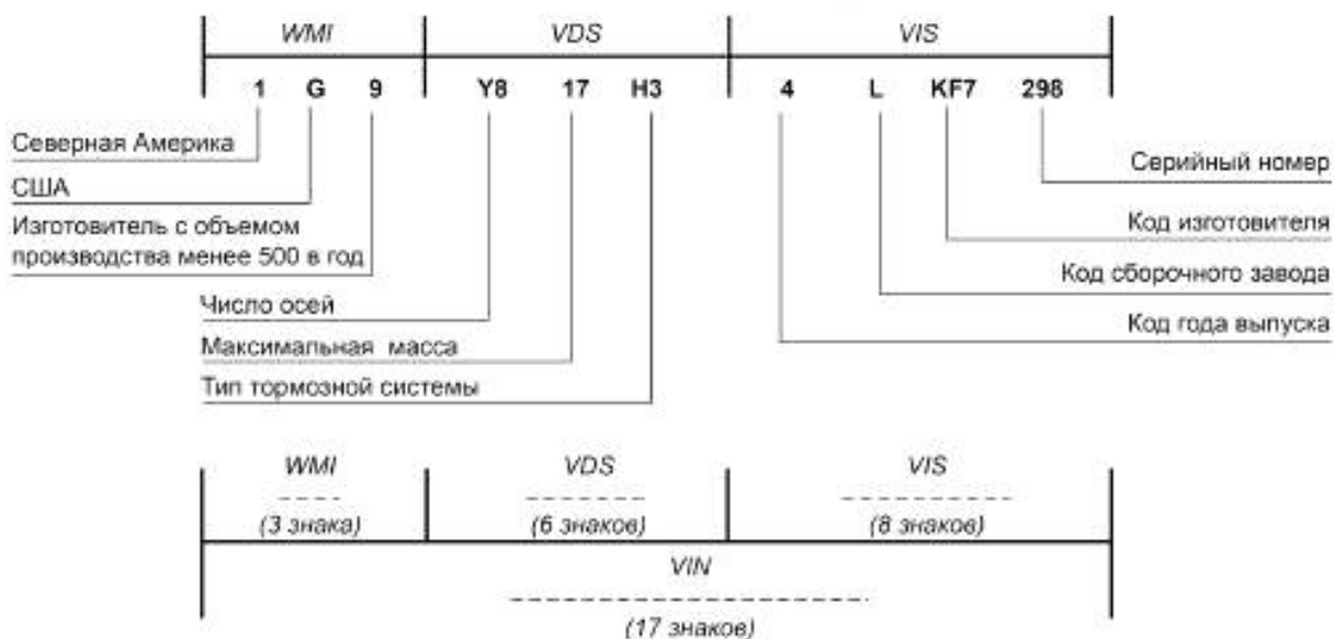
Рисунок Б.2 — Пример № 2 построения кода VIN
