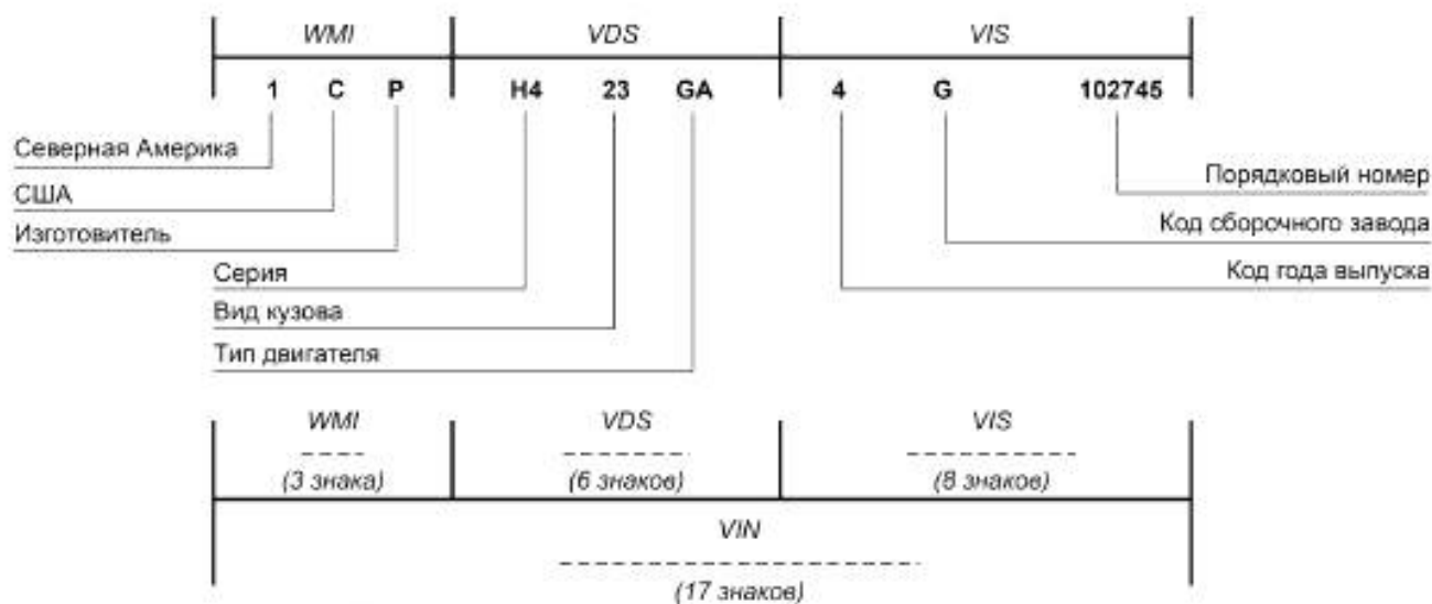
Рисунок Б.1 — Пример № 1 построения кода VIN
