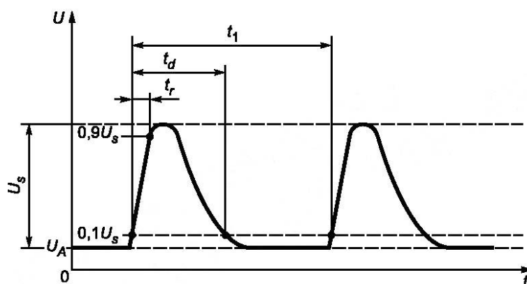
Рисунок 6 — Испытательный импульс 2a
