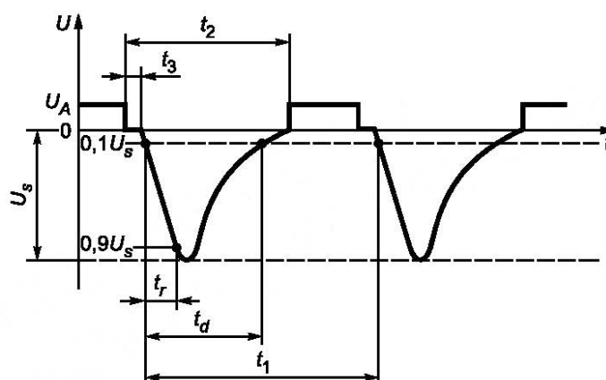
Рисунок 5 — Испытательный импульс 1
