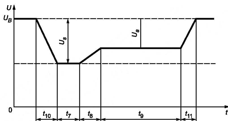
Рисунок 10 — Испытательный импульс 4
