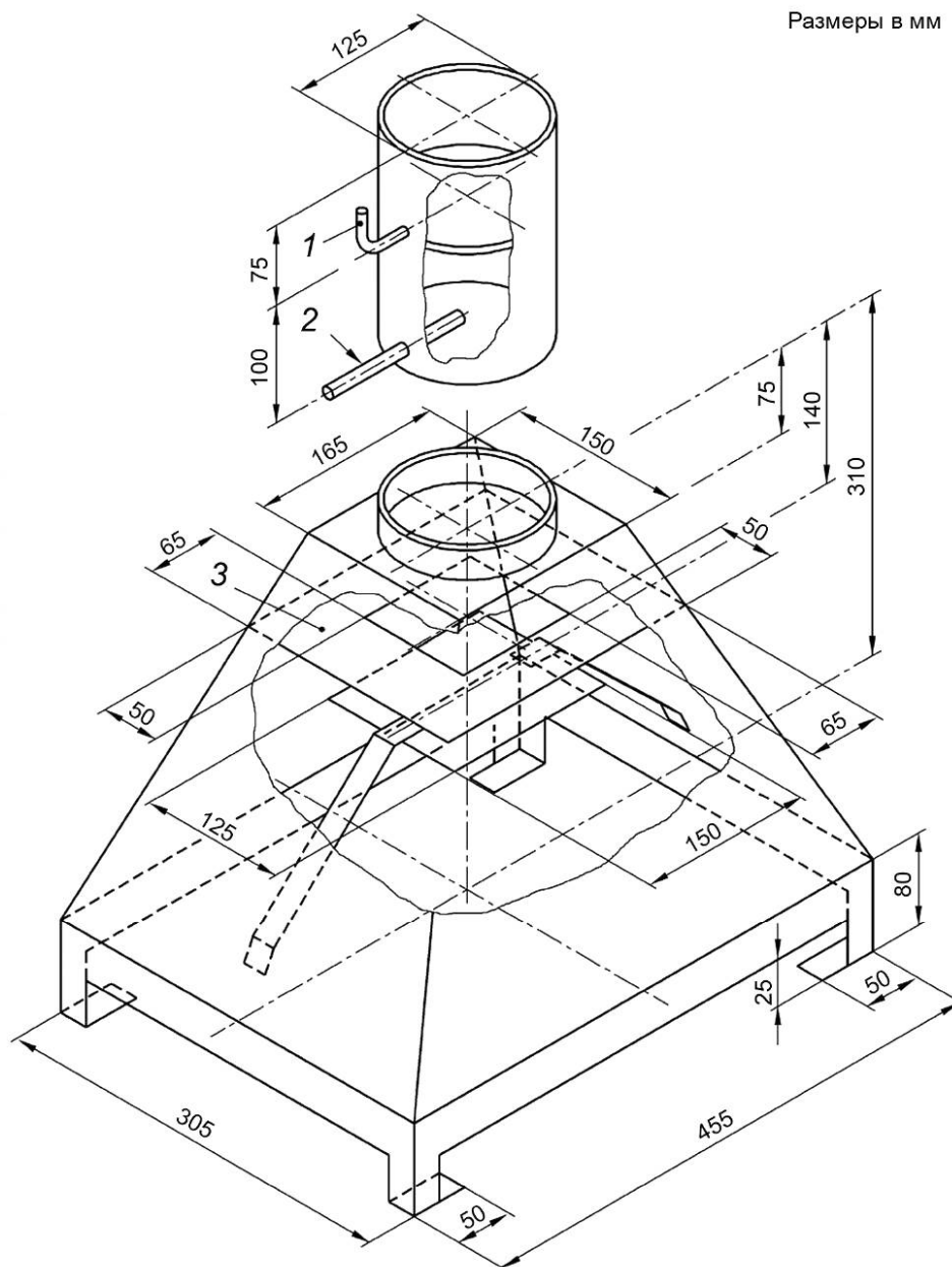
1 — поворотная заслонка; 2 — труба диаметром 8 мм; 3 — кольцеобразный диск
