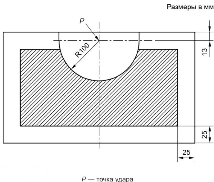
Рисунок G.1 — Точка удара и участок оценки
