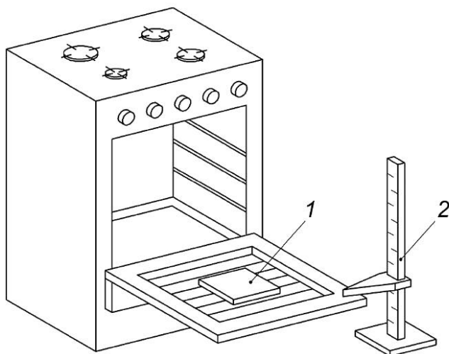
1 — испытательный груз; 2 — измерительное устройство
