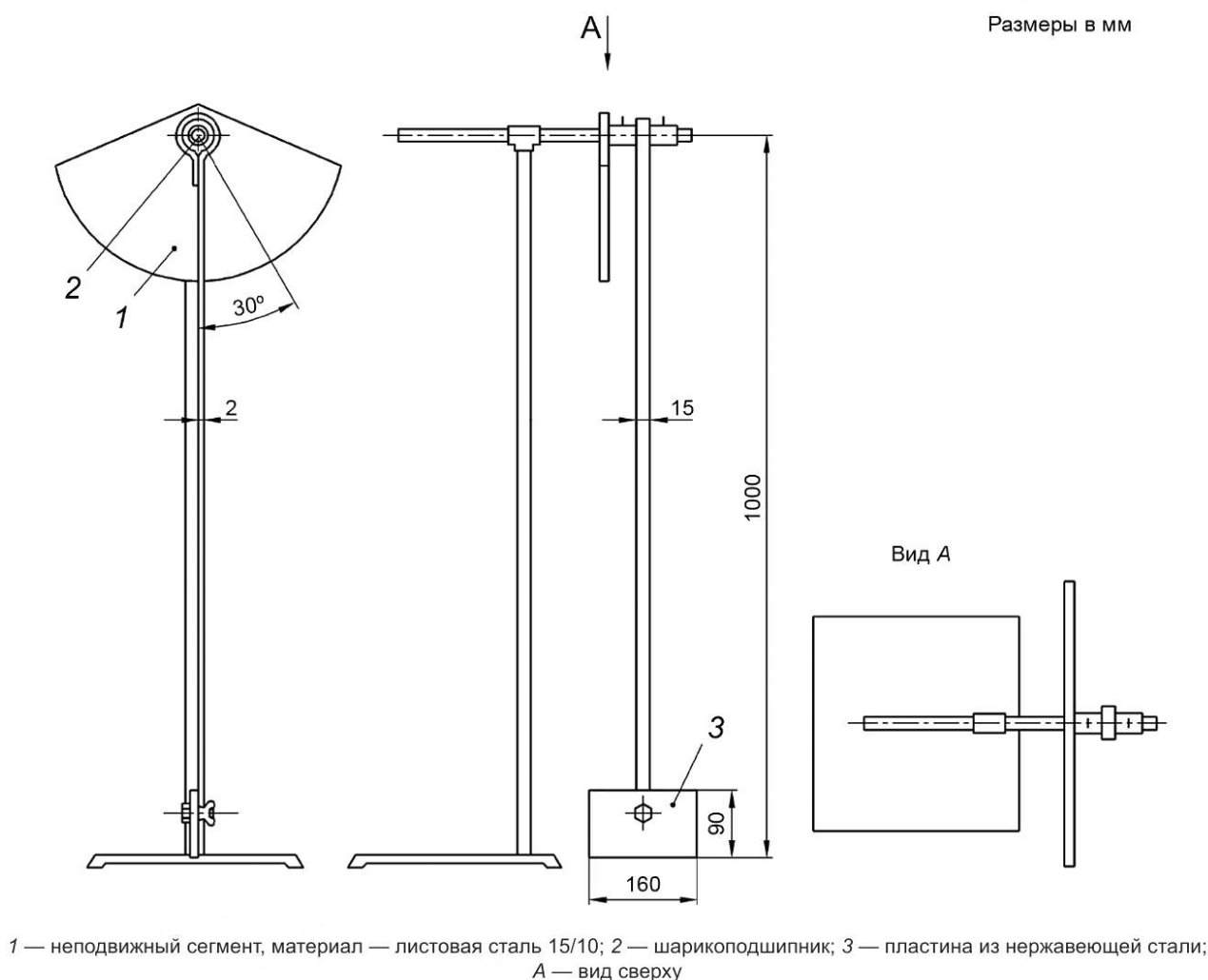
Рисунок 9 — Маятник для испытания сопротивления горелки потоку воздуха
