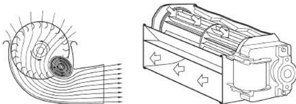
Рисунок 17 — Диаметральный вентилятор
