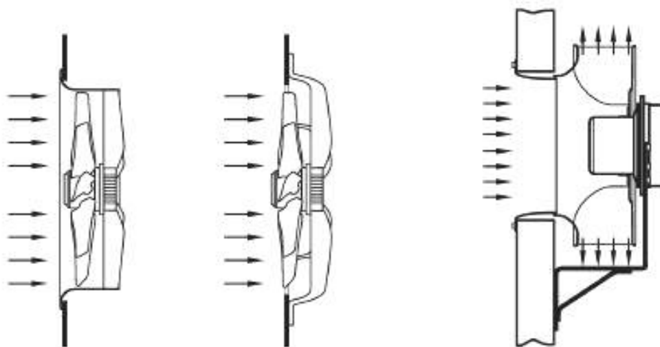
Рисунок 8 — Вентиляторы, встраиваемые в отверстие стены
