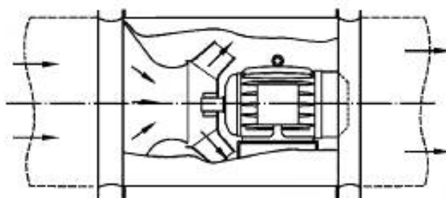
Рисунок 5 — Прямоточный диагональный вентилятор
