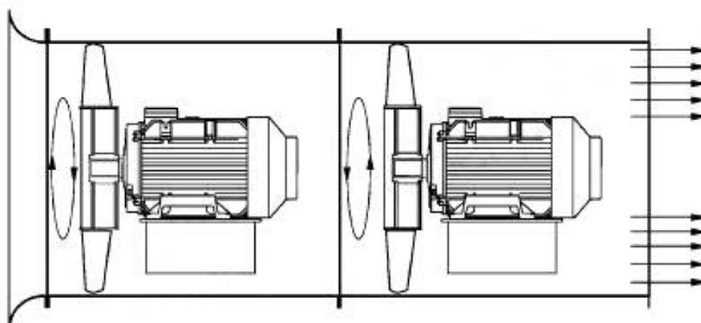
Рисунок 15 — Осевой вентилятор встречного вращения
