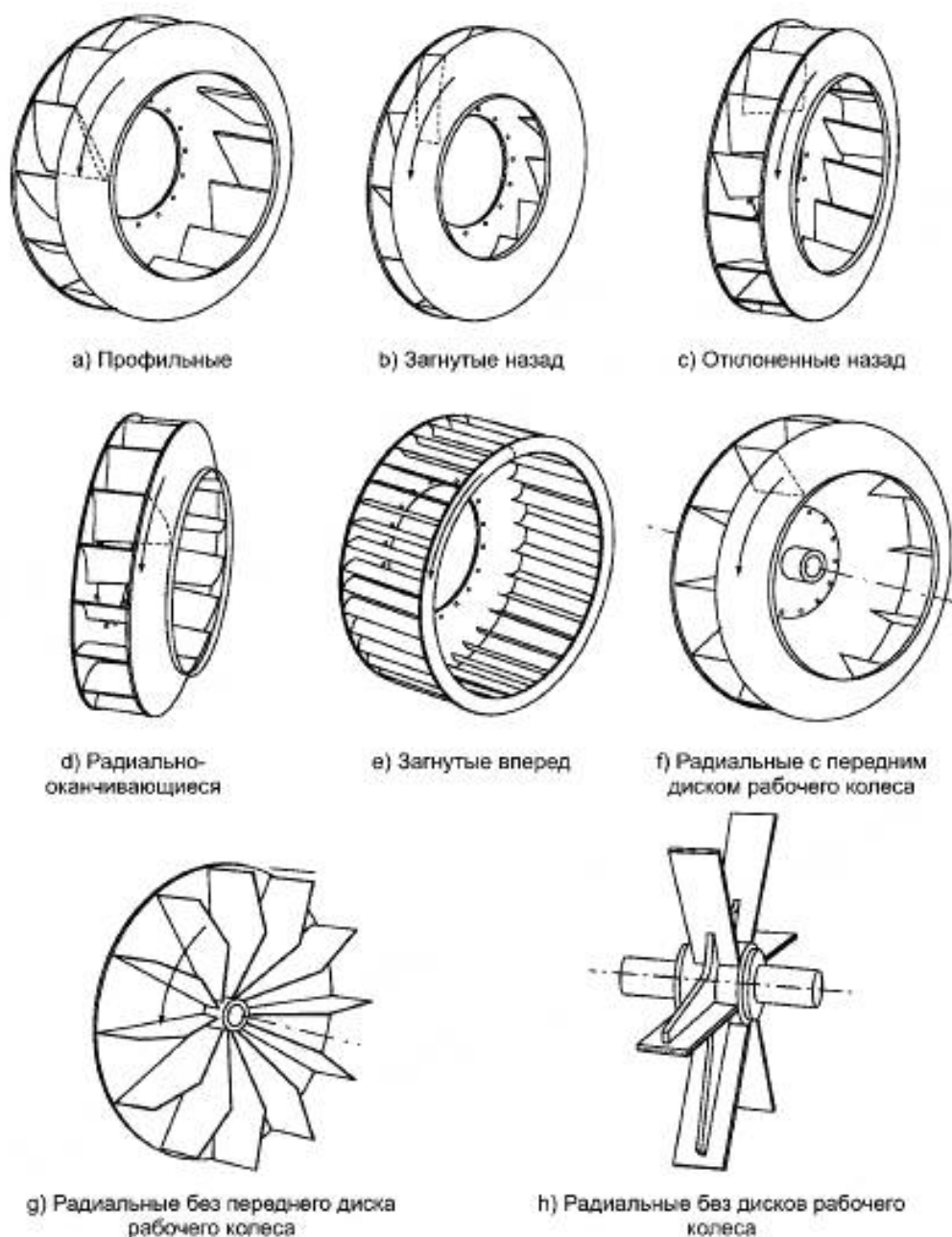
Рисунок 12 — Радиальные рабочие колеса с разными типами лопаток
