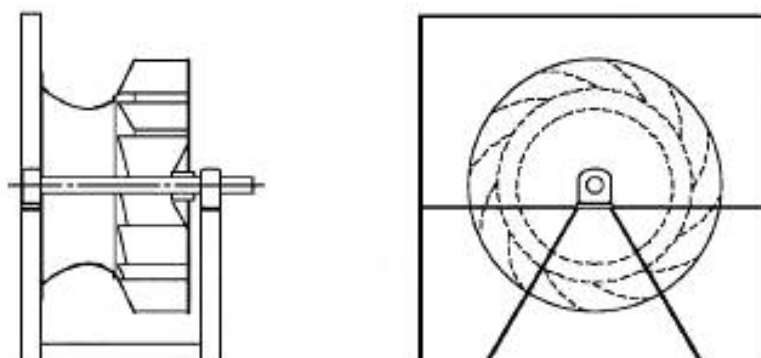
Рисунок 14 — Вентилятор — свободное колесо
