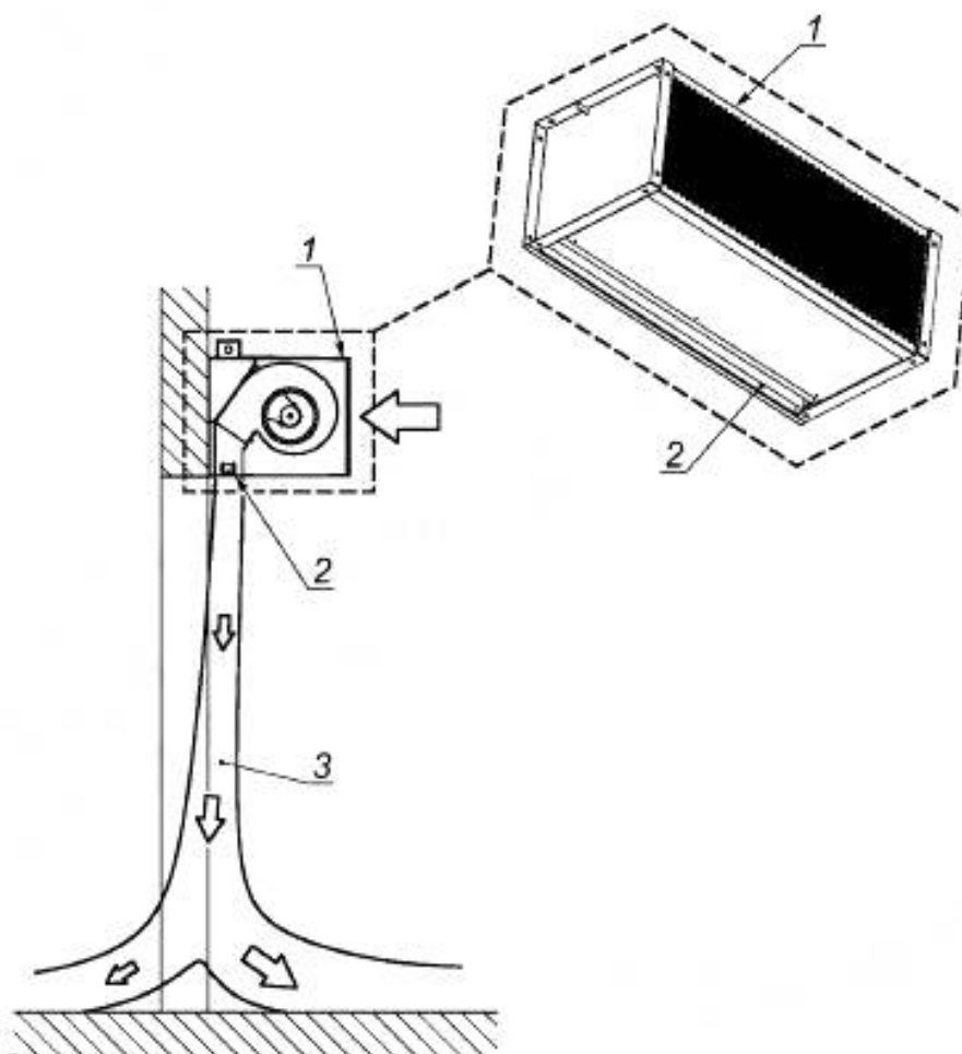
1 — агрегат воздушной завесы; 2 — выходной патрубок; 3 — воздушная завеса
