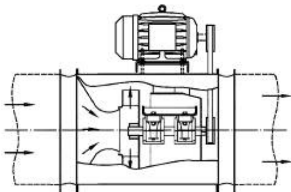
Рисунок 4 — Прямоточный радиальный вентилятор
