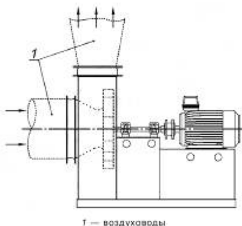
Рисунок 2 — Радиальный вентилятор
