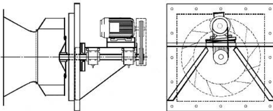
Рисунок 13 — Вентилятор для вентиляторного блока
