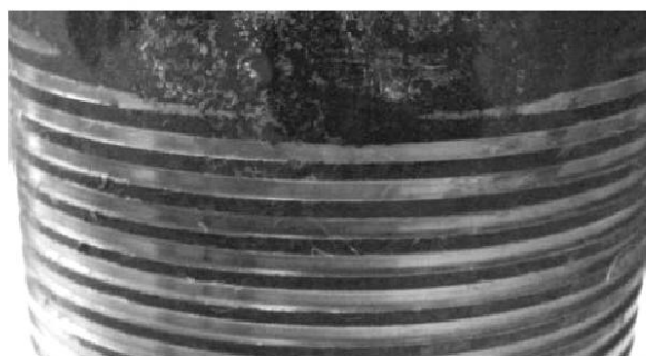
б) Прерванные последние витки перед выходом наружной резьбы
