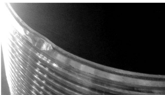
б) Забоина на заходной фаске
