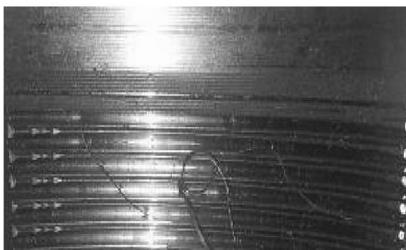
Рисунок 19 — Усы на внутренней резьбе
