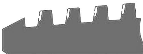
б) Подрез боковой стороны и резьбы вершины витка резьбы
