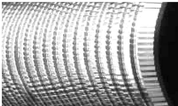
а) Следы вибрации, приводящие к несоответствию геометрических параметров наружной резьбы и заходной фаски
