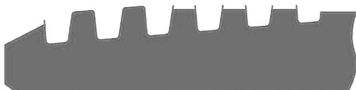
а) Гребни на заходной фаске и вершинах витков наружной резьбы с неполным профилем
