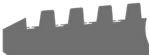
г) Подрез впадины витка резьбы
