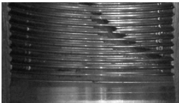
а) Раковина, образовавшаяся на внутренней резьбе после выпадения отслоившегося участка плены
