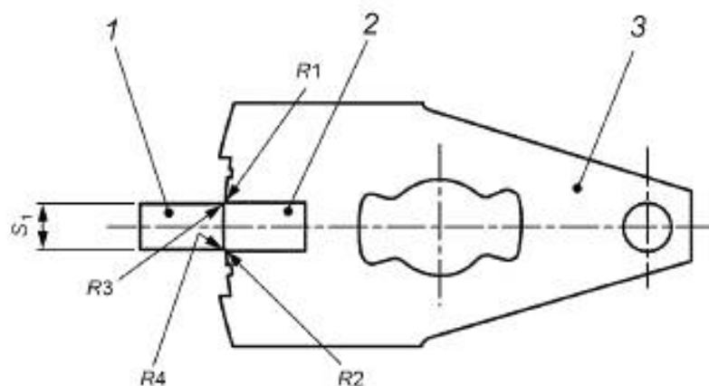
1 — стопорный элемент; 2 — кодовый канал; 3 — сувальда
