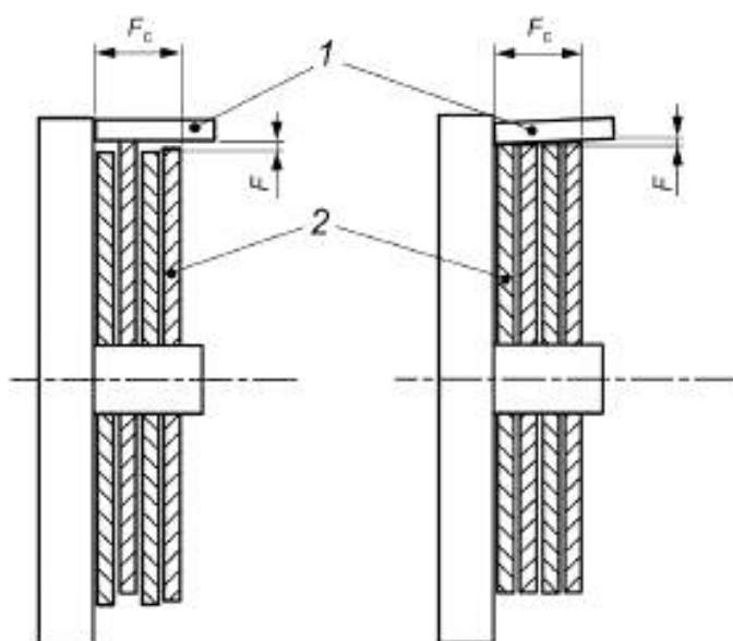
1 — стопорный элемент; 2 — комбинационные диски
