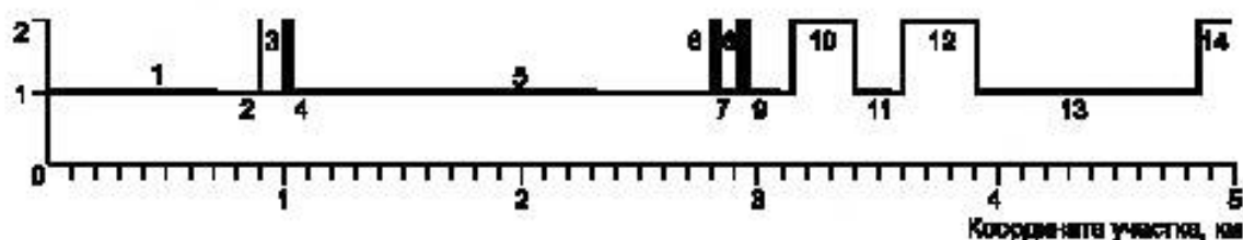
Рисунок Е.5 — Графическая иллюстрация формирования расчетных участков
