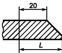
Рисунок 4 — Присоединительный конец под приварку
