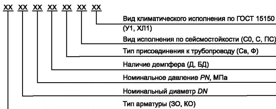
Рисунок 1 — Схема условного обозначения арматуры
