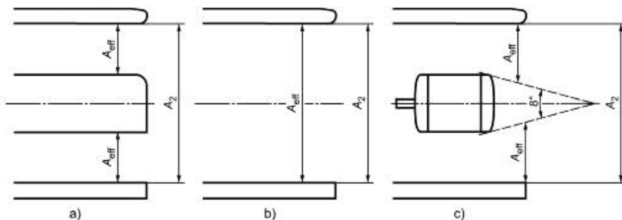
Рисунок 1 — Полная и эффективная площади выхода вентилятора
