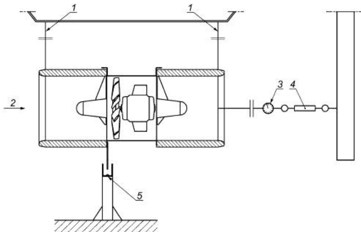
1 — тросы подвески; 2 — направление потока воздуха; 3 — динамометр; 4 — регулируемое крепление; 5 — точка отсчета
