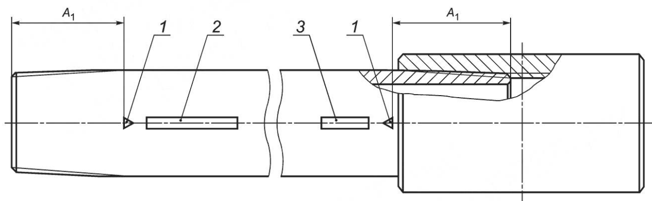
1 — треугольное клеймо; 2 — полоса размером 25 × 610 мм на nipple-конце трубы; 3 — полоса размером 25 × 102 мм на муфтовом конце трубы; A_1 — расстояние от торца трубы до основания треугольного клейма
