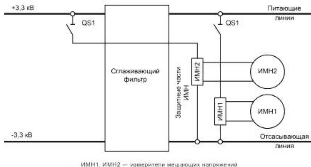
Рисунок 2 — Схема для контроля соответствия требованиям 4.6.1.2, перечисления а) — в)
