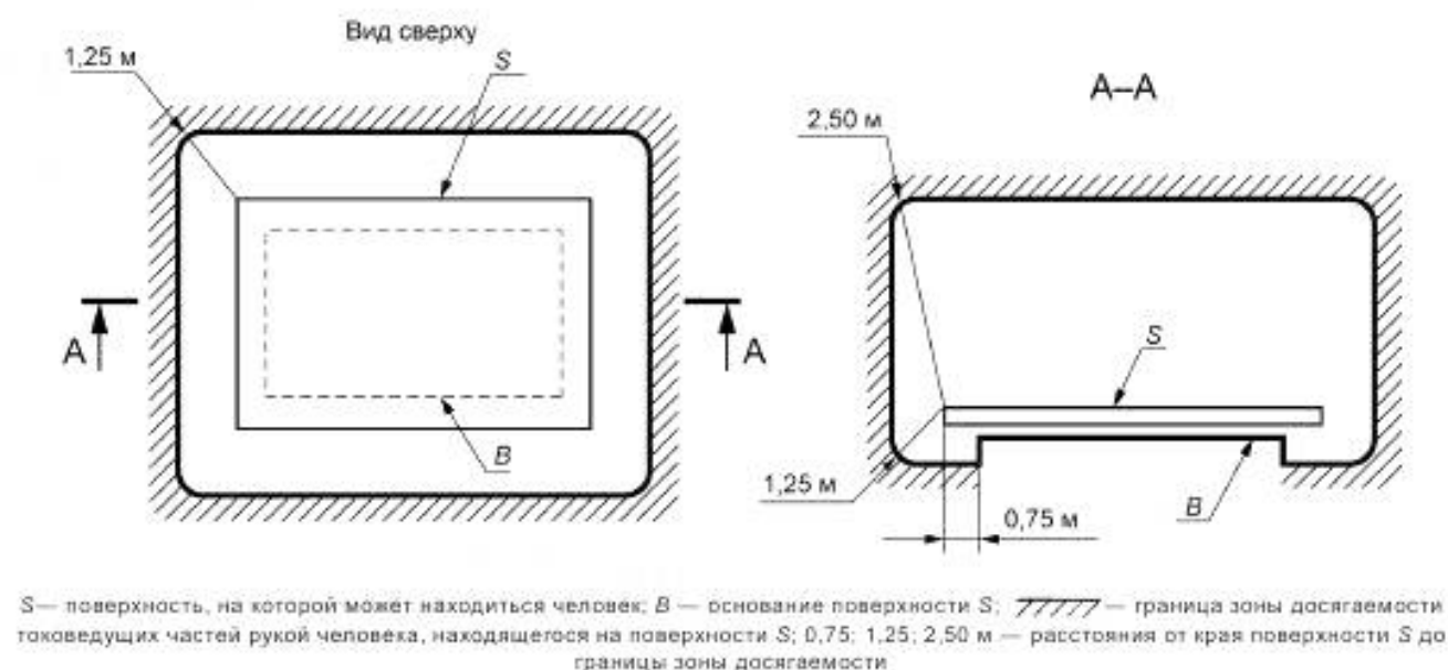
Рисунок 1 — Зона досягаемости в электроустановках напряжением до 1000 В
