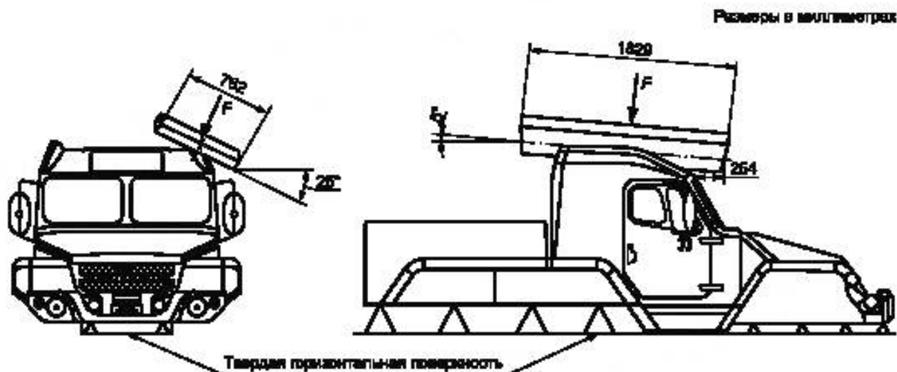
Рисунок 1 — Схема испытания защитных свойств кабины/кузова.
