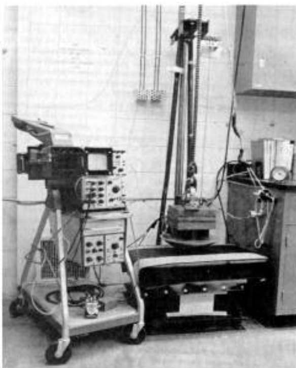
Рисунок 6 — Пример устройства для испытания амортизирующих свойств сиденья
