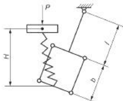
Рисунок 15.1 — Схема шарнирно-сочлененной люльки с вертикальными подвесками
