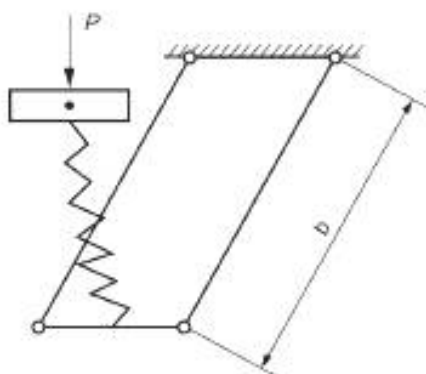
Рисунок 15.2 — Схема однозвенной люлечной подвески
