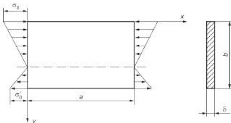
Рисунок 9.1 — Пластина под действием сжатия и изгиба
