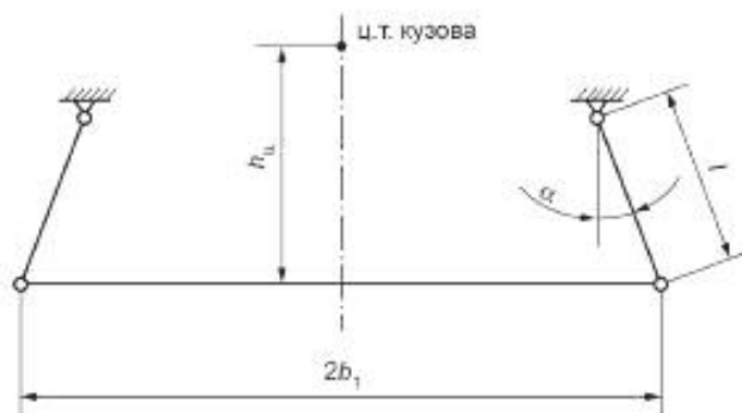
Рисунок 15.3 — Схема люльки с наклонными подвесками
