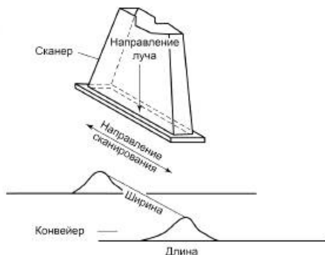
Рисунок 1 — Схема, показывающая длину и ширину сканирующего пучка в конвейерной системе
