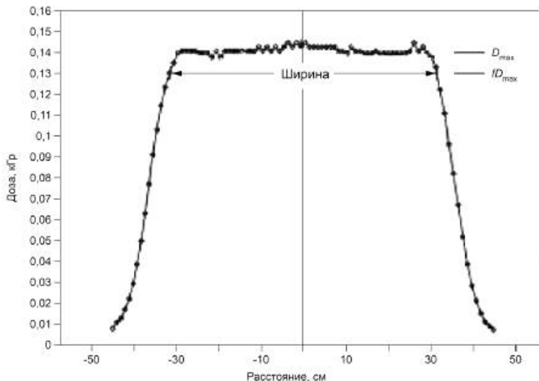
Рисунок 2 — Пример измеренного распределения дозы облучения электронным пучком по ширине пучка, где ширина пучка определена по некоторой заданной доле f от средней максимальной дозы D_{\max}
