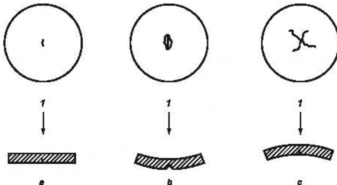
Рисунок 1 — Сечение образцов, поврежденных «трещиной»
