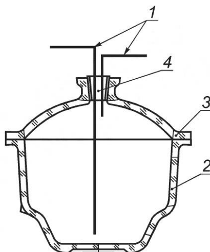
Рисунок А.1 — Стеклянная емкость (экзикатор), имеющая две отводные трубки, используемая для приготовления воздушной вытяжки
