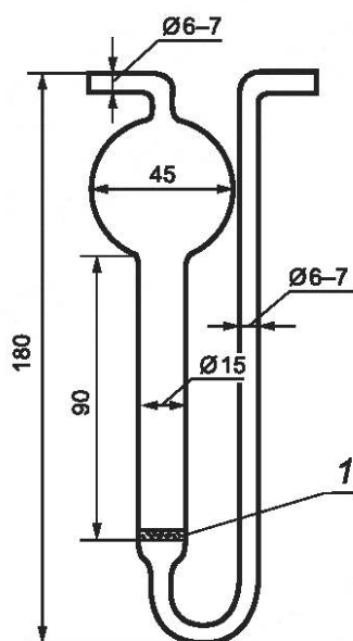
Рисунок А.2 — Поглотитель с пористой стеклянной пластинкой, впаянной в поглотитель
