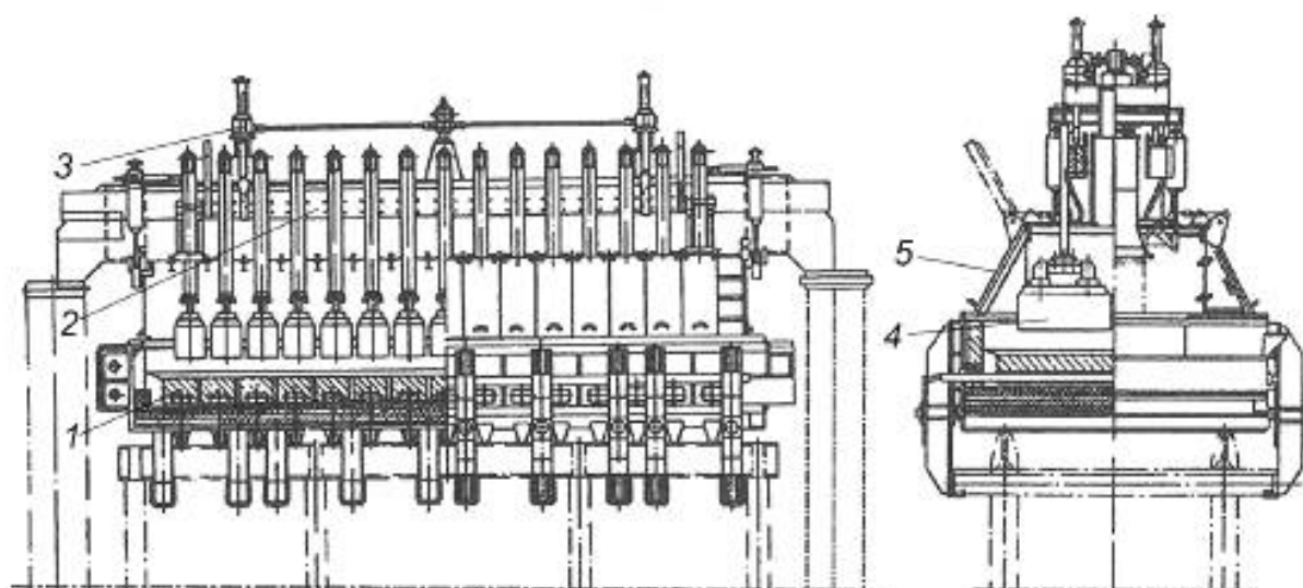
Рисунок 2 — Электролизер ОА
