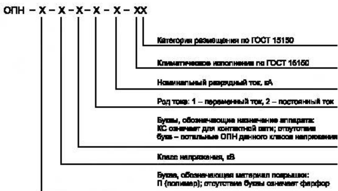
Рисунок 1 — Рекомендуемая структура обозначения ОПН
