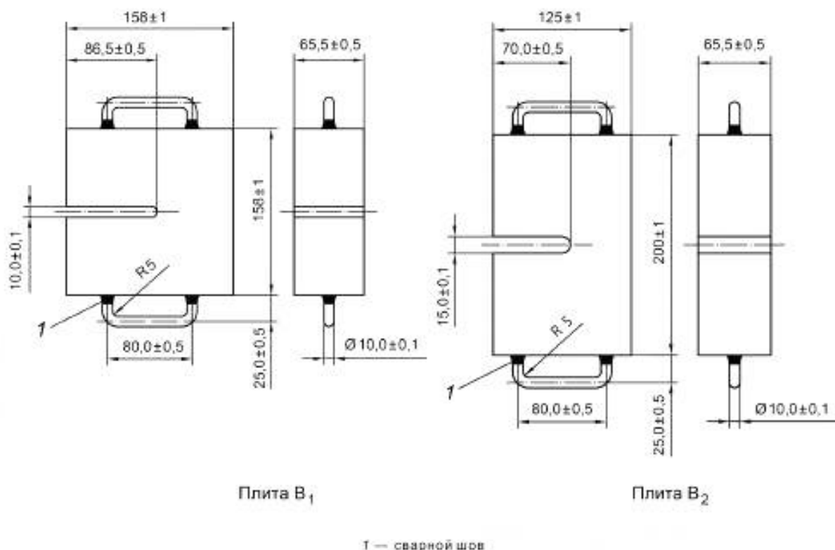
Рисунок 3 — Геометрические размеры плиты В
