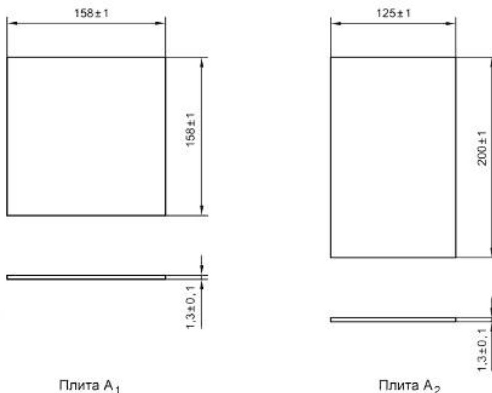
Рисунок 2 — Геометрические размеры плиты А
