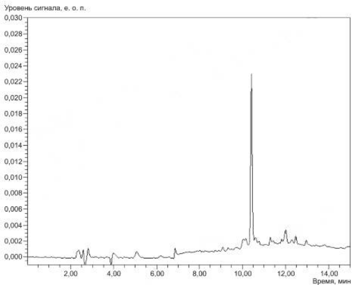
Рисунок Б.2 — Хроматограмма апельсинового сока без СПК
