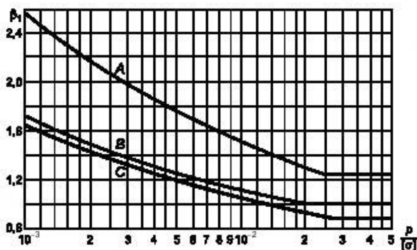
Рисунок 10 — График для определения коэффициента \beta_1
