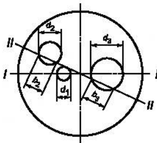
Рисунок 16 — Диаметральные сечения днища или крышки, ослабленные отверстиями
