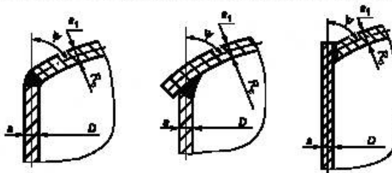
Рисунок 12 — Сферические неотбортованные днища без укрепляющего кольца
