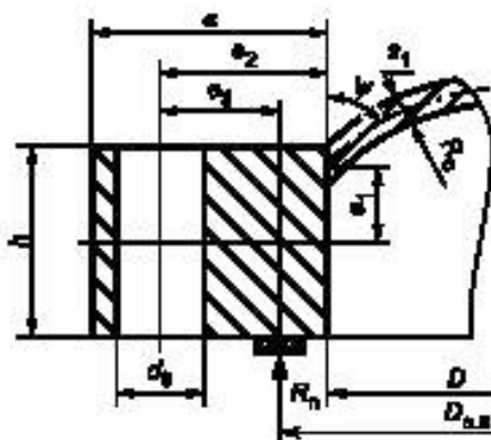
Рисунок 15 — Сферическая неотбортованная крышка
