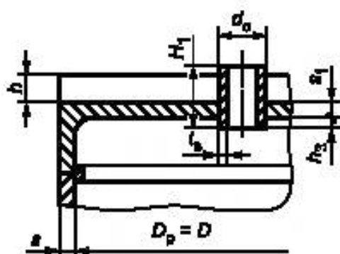
Рисунок 23 — Плоское круглое днище с радиальными ребрами жесткости
