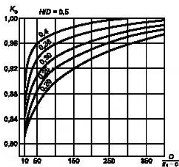
Рисунок 9 — График для определения коэффициента K_3
