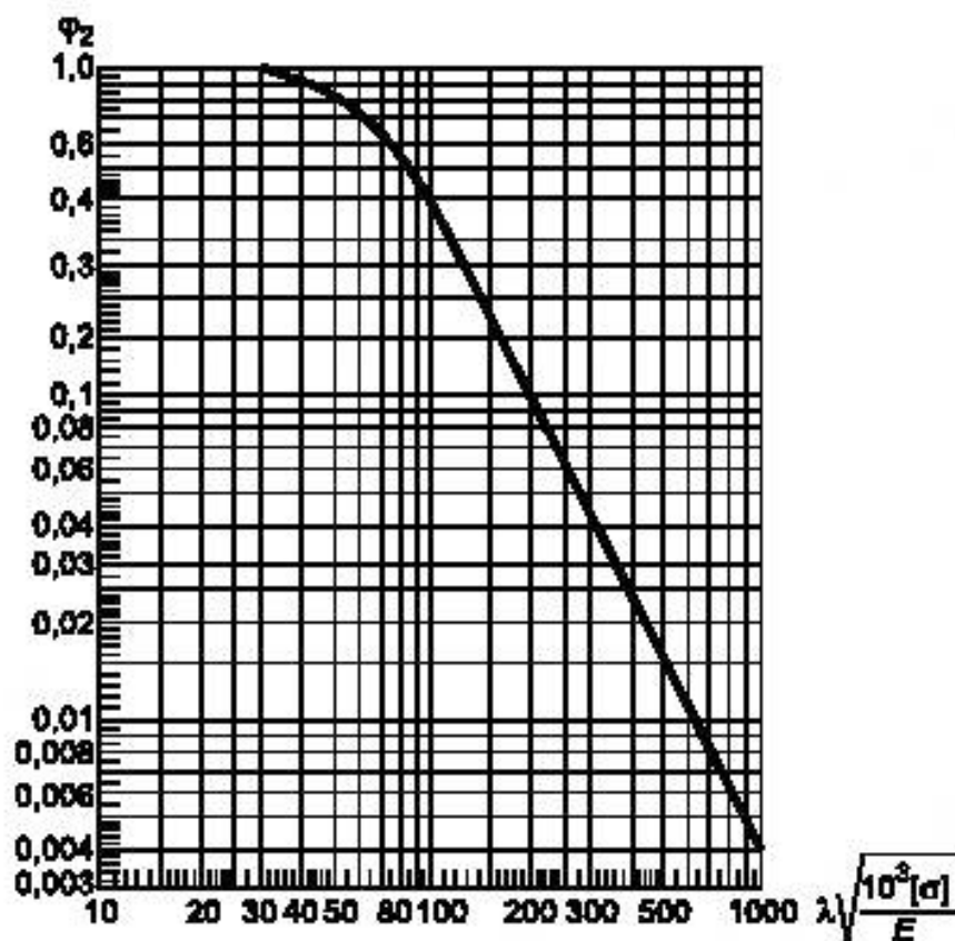
Рисунок 6 — График для определения коэффициента \varphi_2
