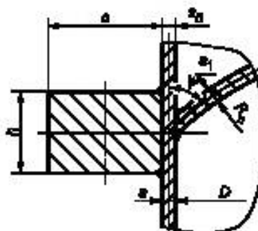
Рисунок 14 — Сферическое неотбортанное днище с кольцом жесткости на обечайке
