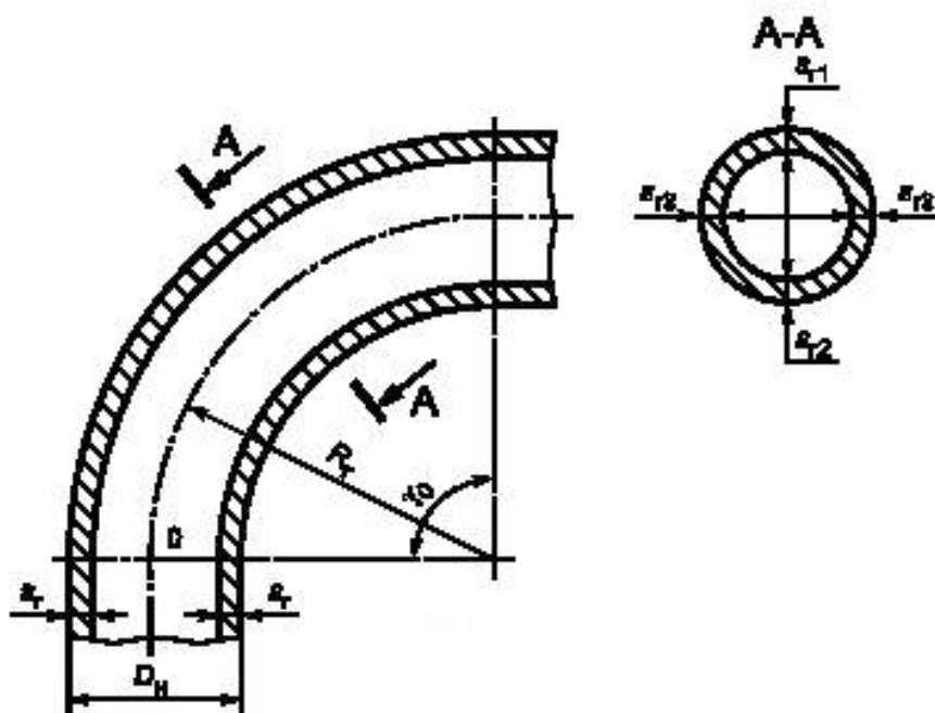
Рисунок А.1 — Отвод (колено)
