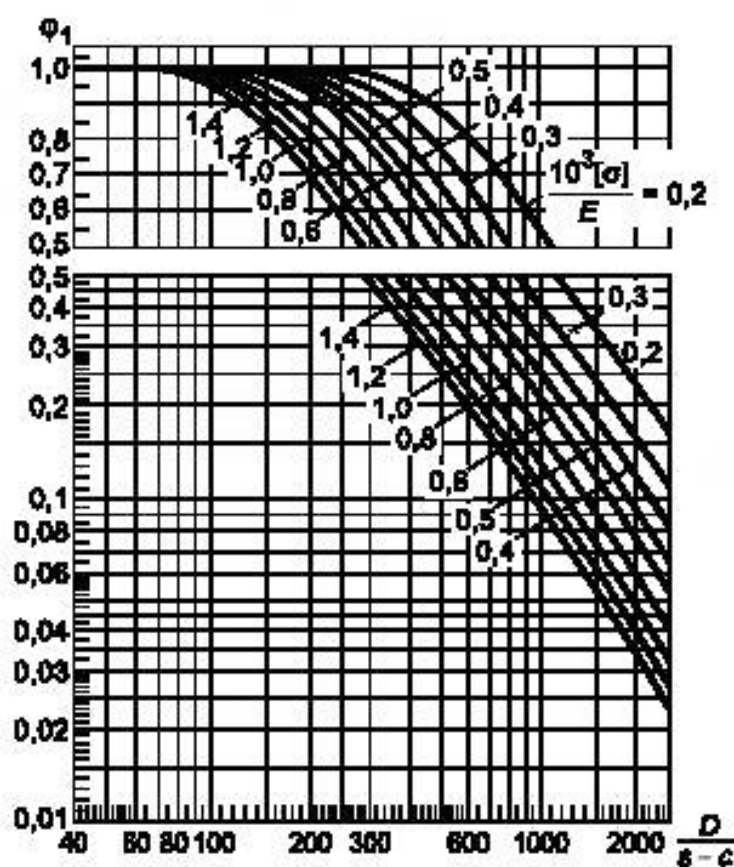
Рисунок 5 — График для определения коэффициента \varphi_1
