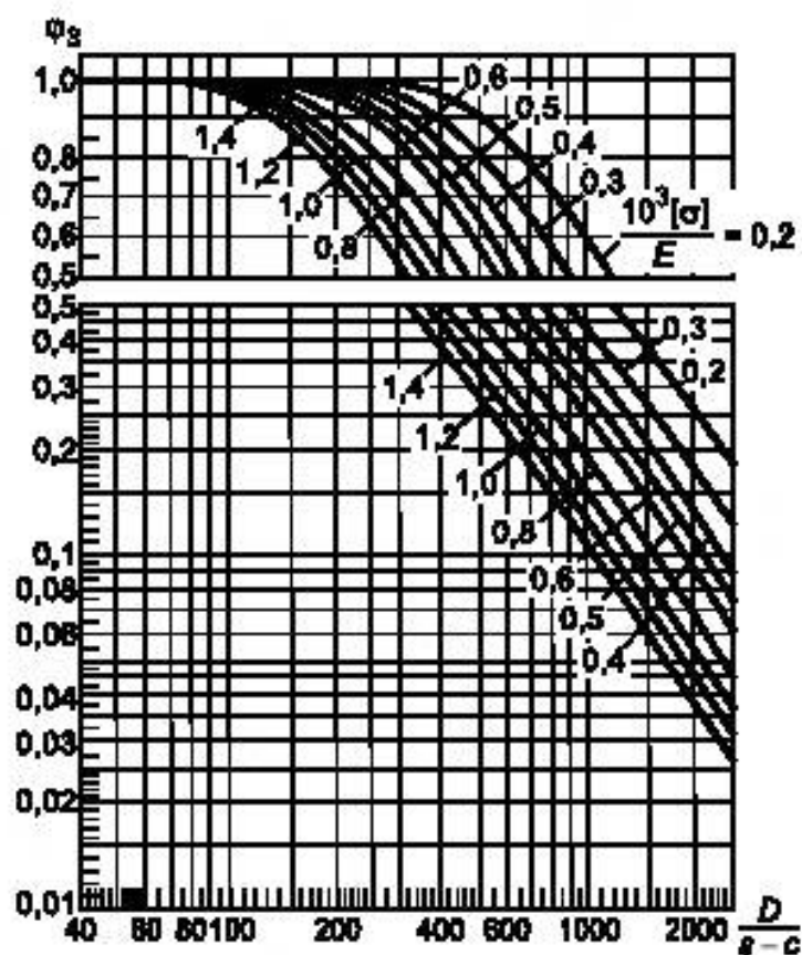
Рисунок 7 — График для определения коэффициента \varphi_3
