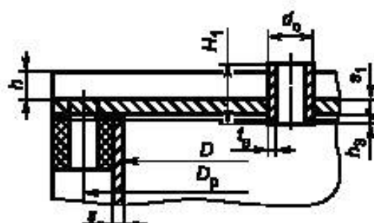
Рисунок 22 — Плоская круглая крышка с радиальными ребрами жесткости
