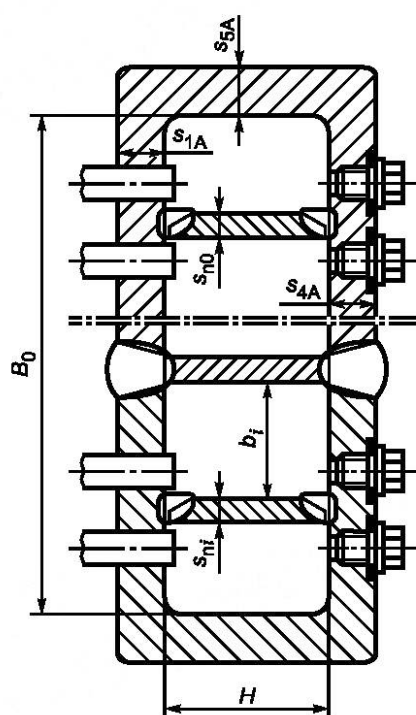
Рисунок 24 — Штампованная камера с перегородками
