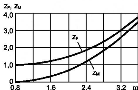
Рисунок 19 — Коэффициенты z_F и z_M
