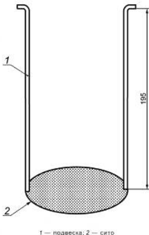
Рисунок 1 — Сито с подвеской
