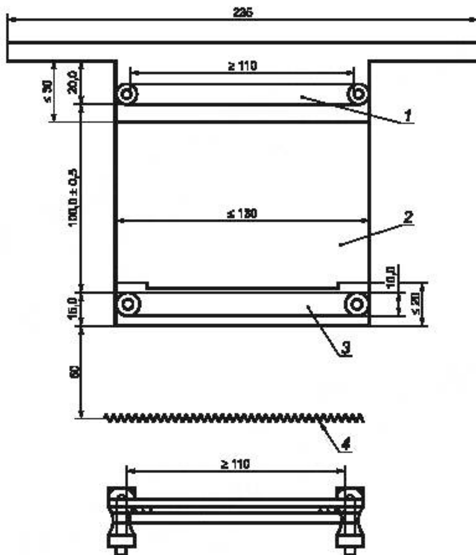
1 — верхний зажим; 2 — образец; 3 — нижний зажим; 4 — сито
