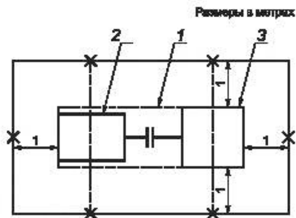
а) Медианная плоскость измерительной поверхности
