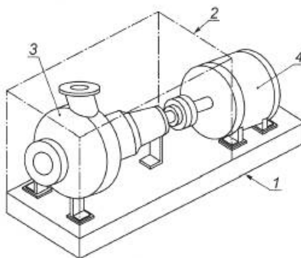
1 — звукоотражающая плоскость; 2 — огибающий параллелепипед; 3 — насос; 4 — привод
