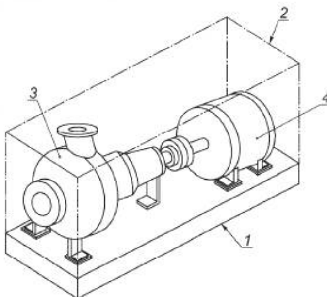
1 — звукоотражающая плоскость; 2 — огибающий параллелепипед; 3 — насос; 4 — привод
