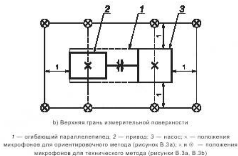
Рисунок В.3 — Положения микрофонов
