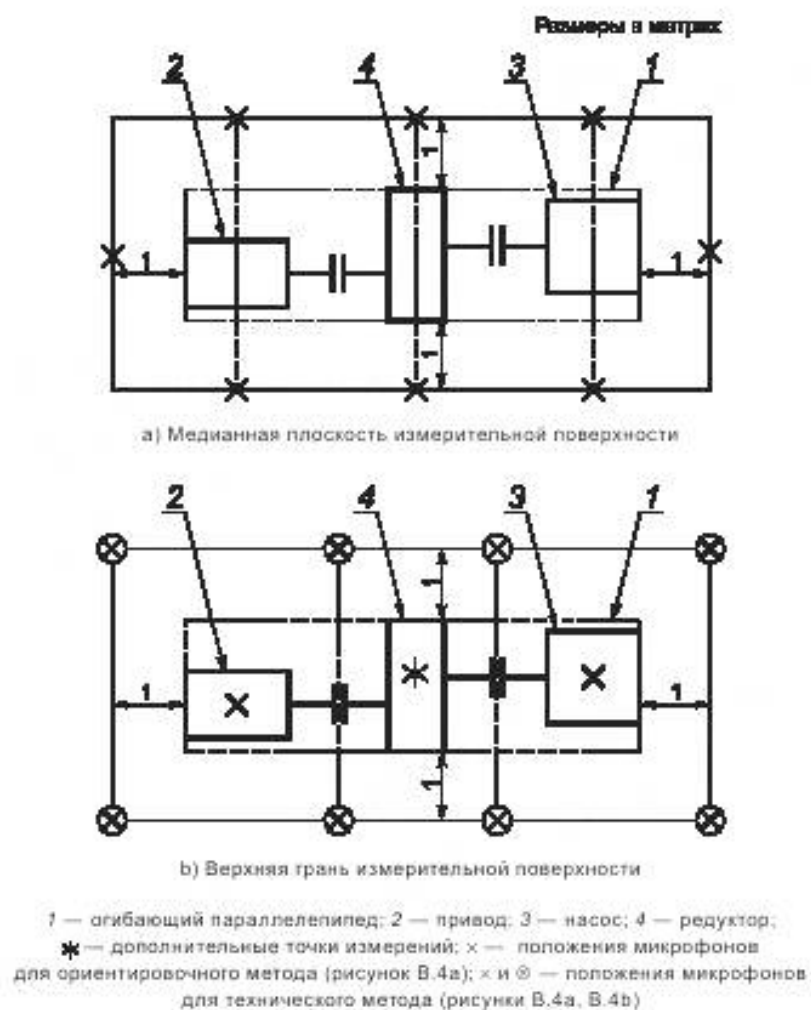
Рисунок В.4 — Положения микрофонов
