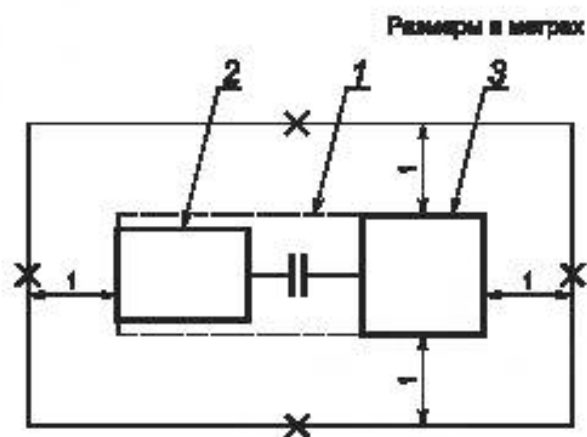
а) Меряющая плоскость измерительной поверхности
