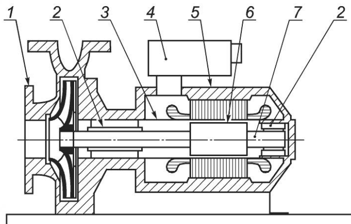
1 — гидравлическая часть; 2 — подшипник; 3 — гильза (вкладыш); 4 — кабельный ввод; 5 — сборка статора; 6 — защитный слой «беличья клетка»; 7 — ротор
