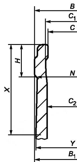
Рисунок В.2 — Сечение венчика горловины бутылки
