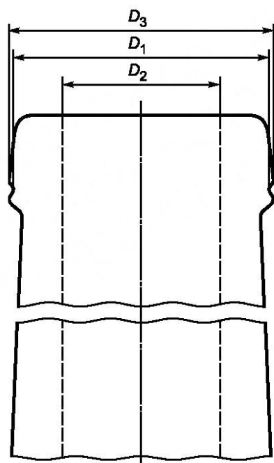
Рисунок В.1 — Венчик горловины бутылки
