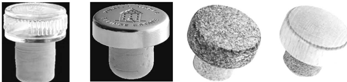
Рисунок А.4 — Составная пробка Т-образной формы с приклеенным фланцем
