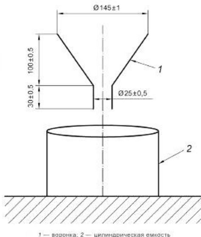
Рисунок 1 — Геометрические параметры воронки
