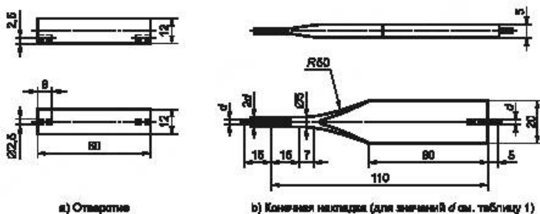
Рисунок 6 — Алюминиевый шаблон
