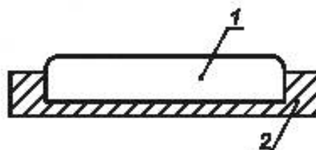
1 — смола; 2 — форма
