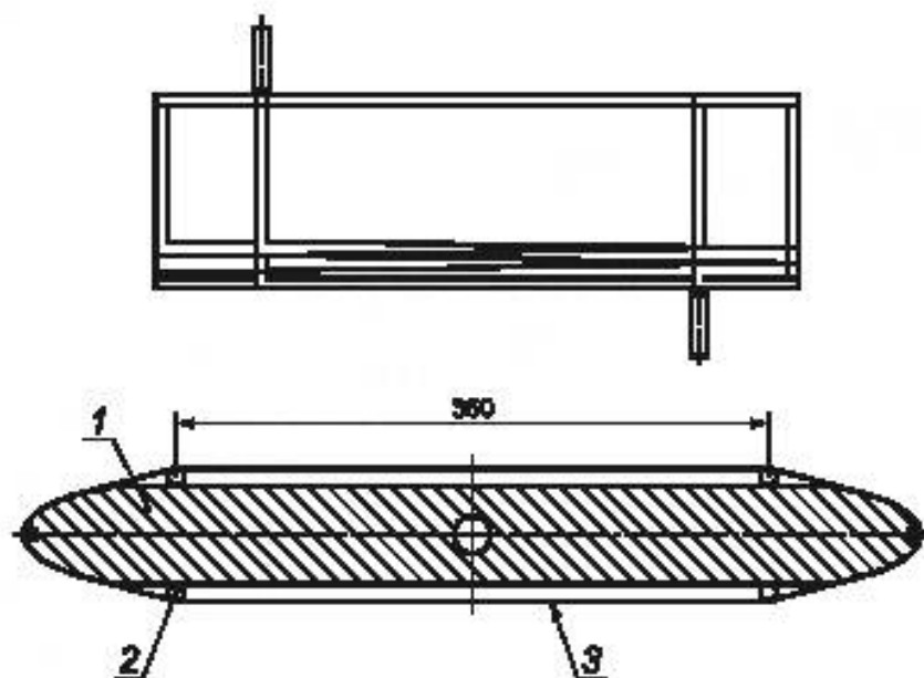
1 — оправка; 2 — силиконовые стержни диаметром 5 мм; 3 — пропитанный ровинг
