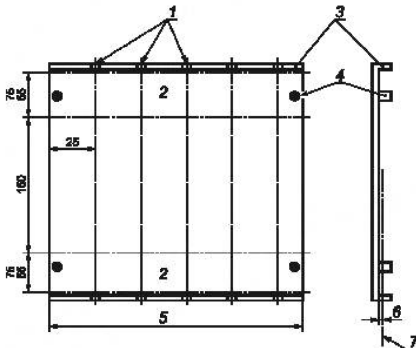
1 — прорезы для ровингов; 2 — полосы картона или композита; 3 — стенка; 4 — проставки; 5 — размеры зависят от количества образцов; 6 — толщина картона или композита; 7 — уровень нижнего края надрезов
