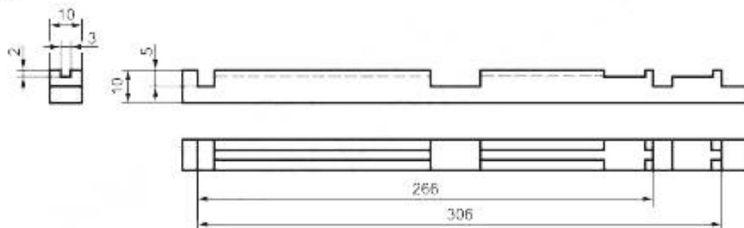
Рисунок 8 — Шаблон для вырезки образцов из пропитанного ровинга
