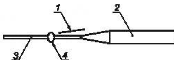
1 — лезвие бритвы; 2 — накладка; 3 — пропитанный ровинг; 4 — обрезаемый облой
