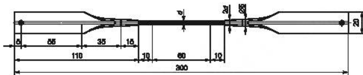
Рисунок 4 — Образец
