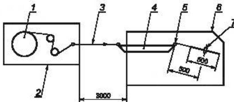
1 — бобина ровинга или паковка; 2 — шпулярник, оборудованный натяжителями; 3 — ровинг; 4 — ванна для пропитки; 5 — фильера; 6 — намоточный станок; 7 — оправка
