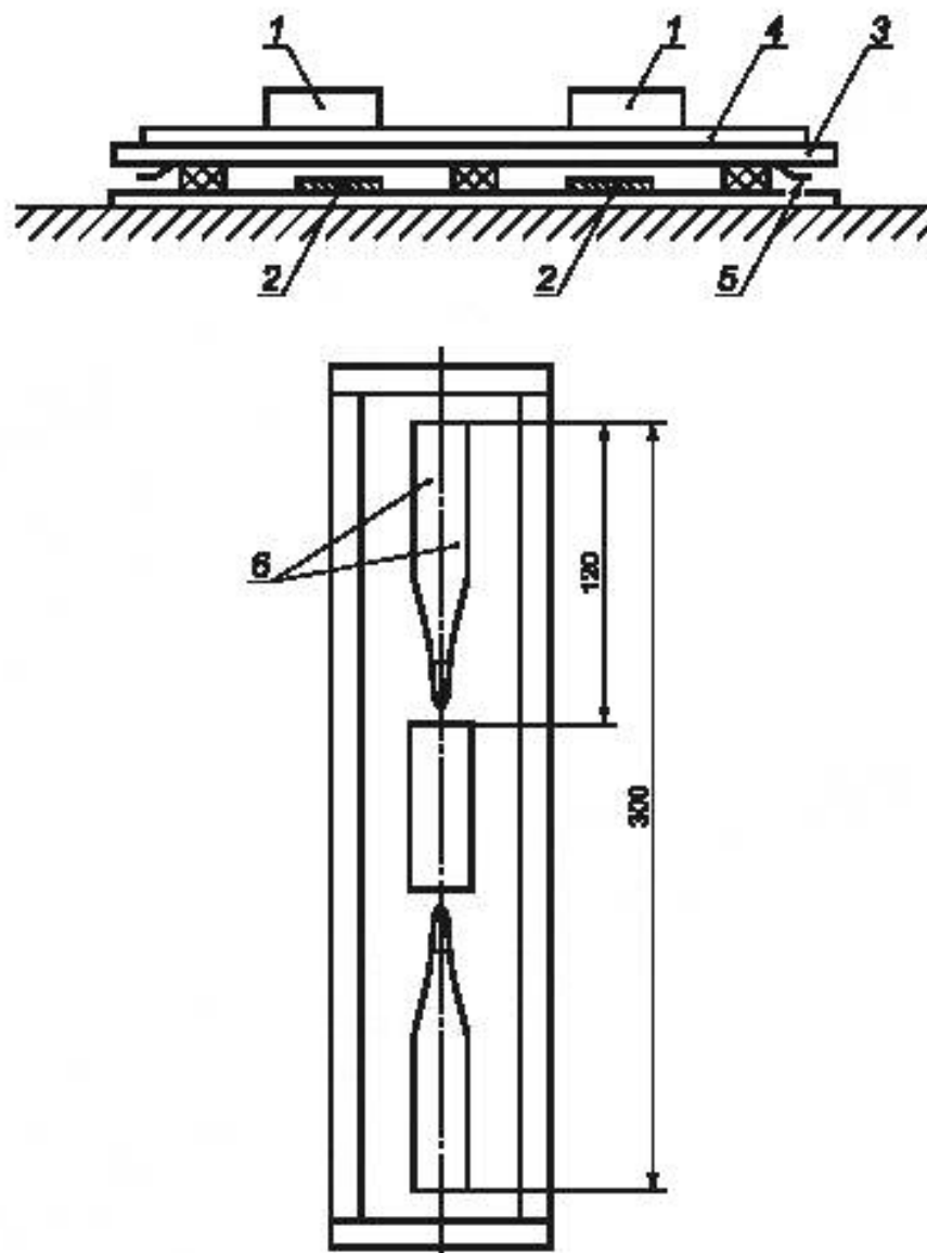
Рисунок 5 — Оборудование для изготовления формы
