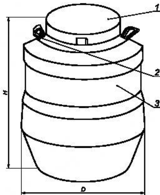
Рисунок А.8 — Фляга ФЛ I-1
