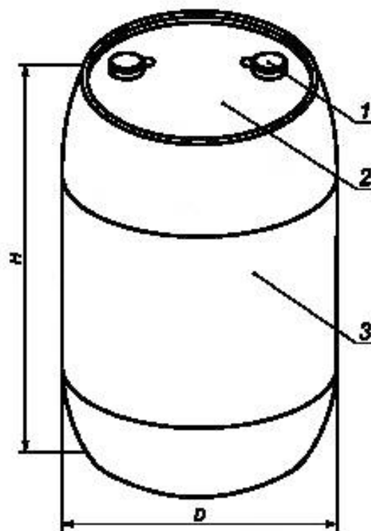
Рисунок А.7 — Бочка БЧ I-4
