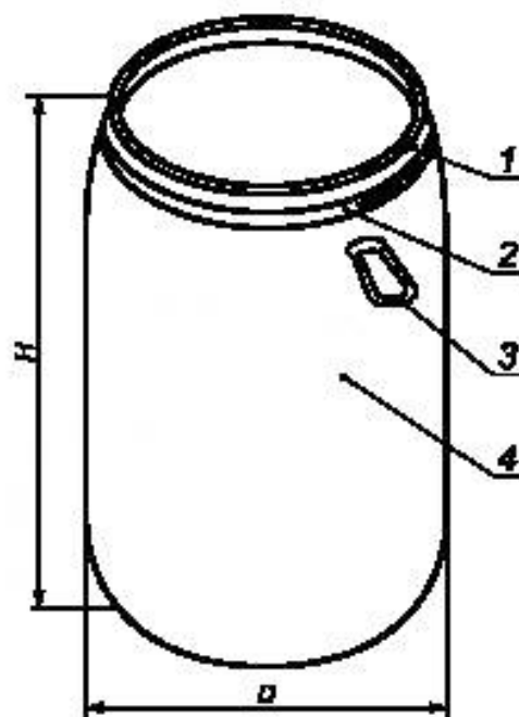
Рисунок А.5 — Бочка БЧ I-2
