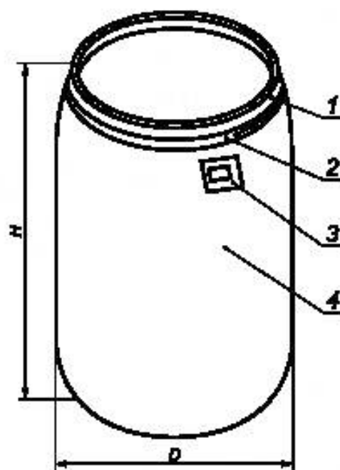
Рисунок А.6 — Бочка БЧ I-3
