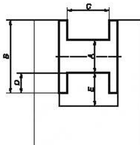
Рисунок 1 — Схема к определению основных размеров барабана лебедки*
