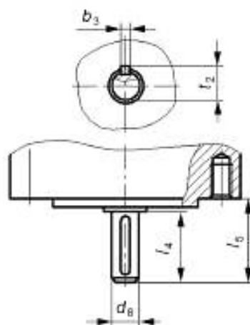
Рисунок 9 — Ведущие подвижные детали группы D
