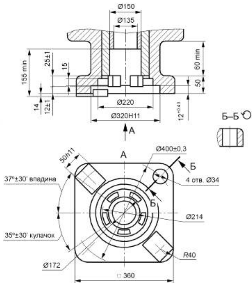
Рисунок А.13 — Присоединение привода типа Д
