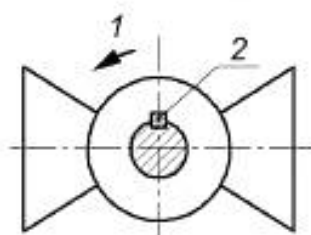
Рисунок 12 — Положение одной шпонки на шпинделе закрытой арматуры
