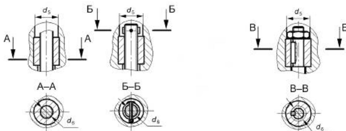
Рисунок 4 — Ведущая подвижная деталь группы А
