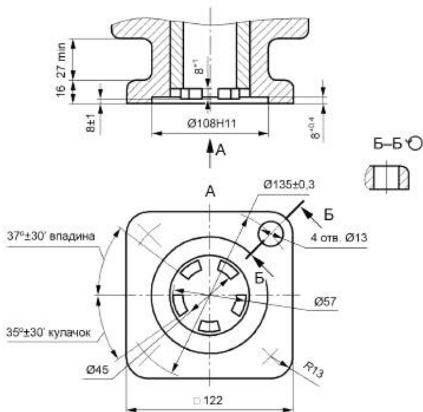
Рисунок А.9 — Присоединение привода типа Б
