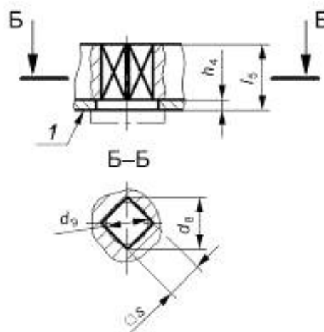
Рисунок 15 — Соединение с диагональной квадратной головкой
