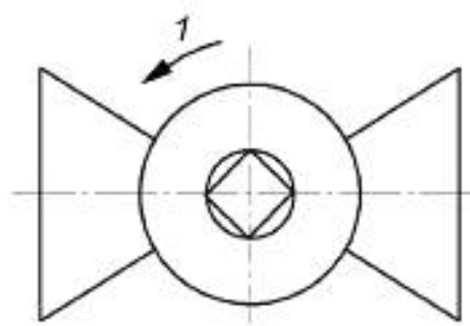
Рисунок 17 — Положение диагональной квадратной головки на закрытой арматуре
