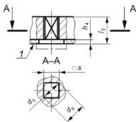
Рисунок 14 — Соединение с параллельной квадратной головкой
