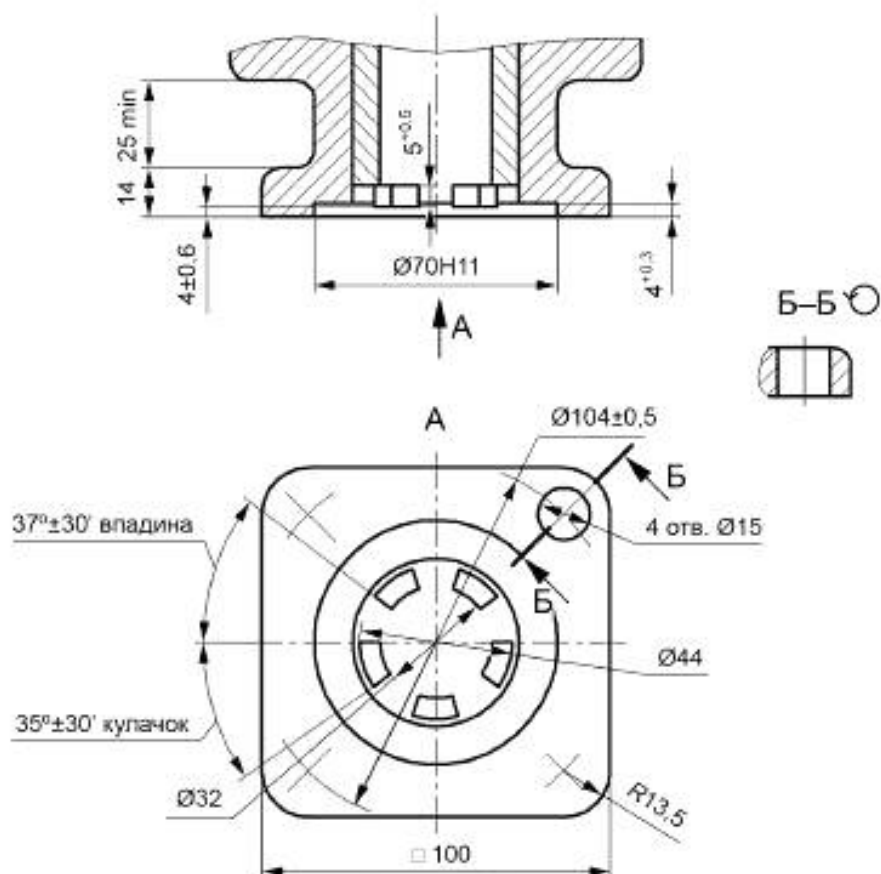
Рисунок А.7 — Присоединение привода типа АК
