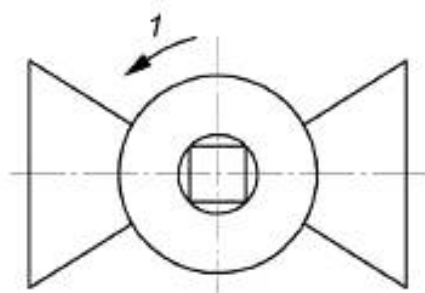
Рисунок 16 — Положение параллельной квадратной головки на закрытой арматуре
