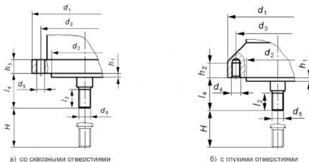
Рисунок 10 — Ведущие подвижные детали линейного привода
