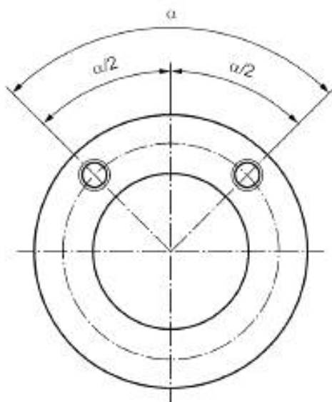
Рисунок 3 — Расположение отверстий для типов присоединений F03—F100
