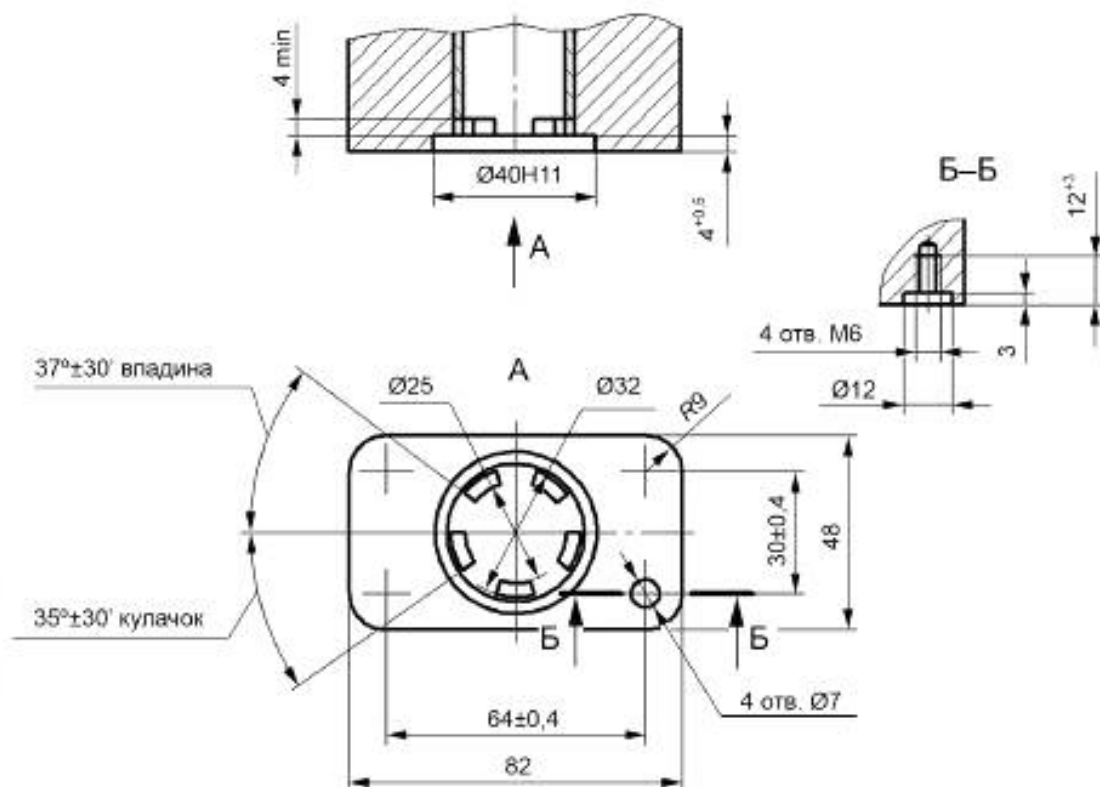
Рисунок А.3 — Присоединение привода типа МК
