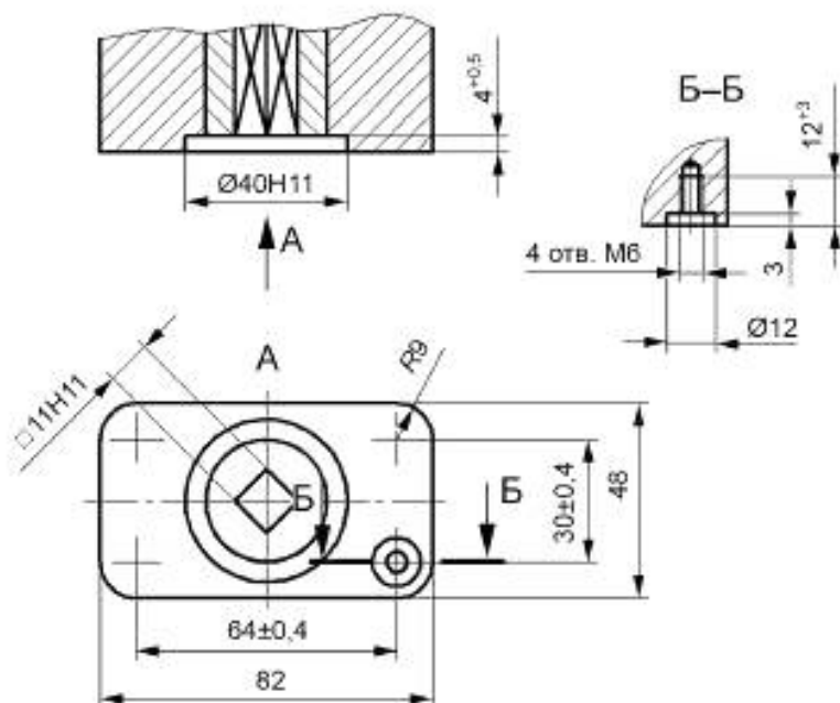
Рисунок А.1 — Присоединение привода типа МЧ
