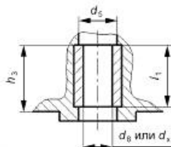
Рисунок 4 — Ведущая подвижная деталь группы А
