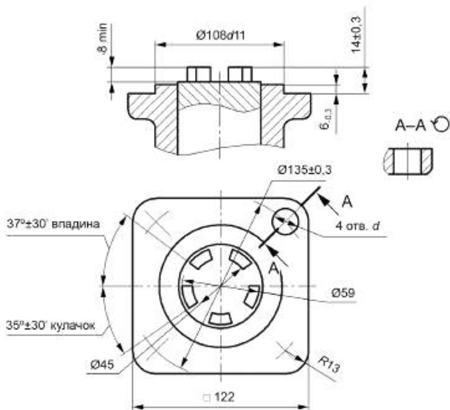
Рисунок А.9 — Присоединение привода типа Б
