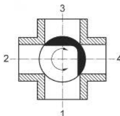
Рисунок А.19 — Ходы 1 и 2 соединены, ходы 3 и 4 закрыты
