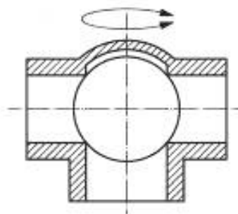
Рисунок А.2 — Вертикальный тип
