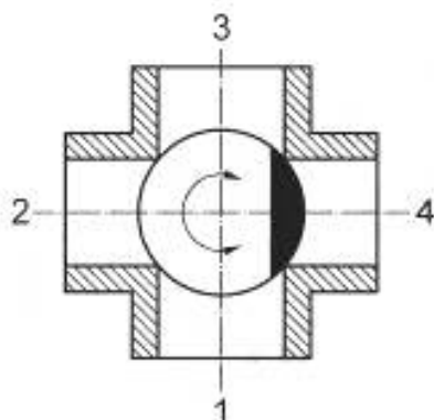
Рисунок А.18 — Ходы 1, 2 и 3 соединены, ход 4 закрыт
