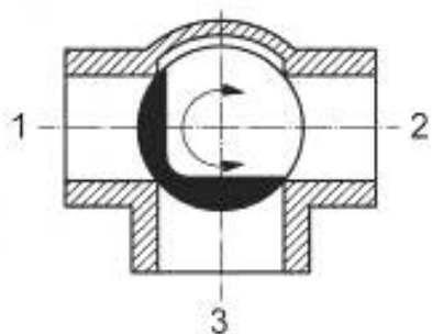
Рисунок А.12 — Кран закрыт
