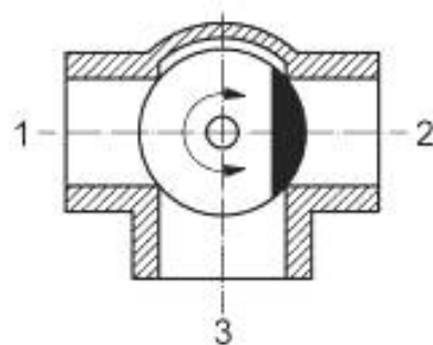
Рисунок А.17 — Ход 2 закрыт, ходы 1 и 3 соединены
