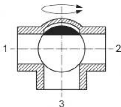
Рисунок А.9 — Ходы 1, 2 и 3 соединены
