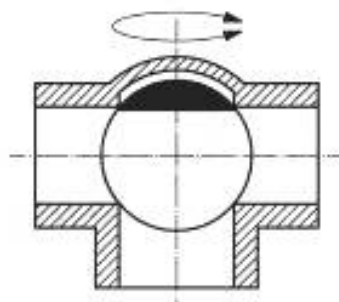
Рисунок А.6 — Горизонтальный тип, Т-образное отверстие
