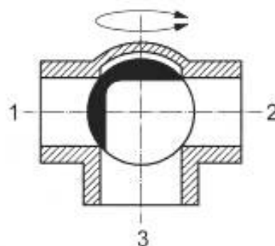
Рисунок А.8 — Ходы 2 и 3 соединены, ход 1 закрыт
