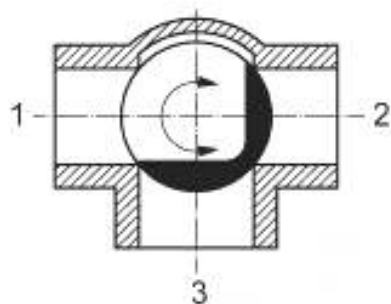
Рисунок А.13 — Кран закрыт
