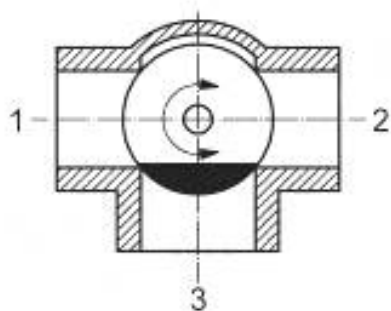
Рисунок А.16 — Ход 3 закрыт, ходы 1 и 2 соединены
