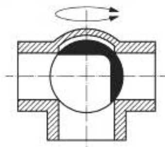
Рисунок А.4 — Вертикальный тип, L-образное отверстие
