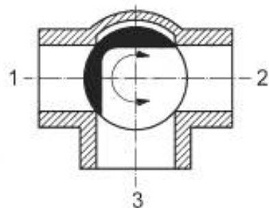
Рисунок А.11 — Ход 1 закрыт, ходы 2 и 3 соединены
