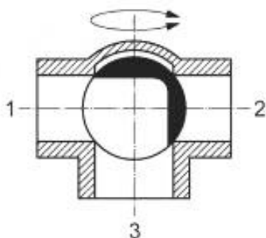
Рисунок А.7 — Ходы 1 и 3 соединены, ход 2 закрыт
