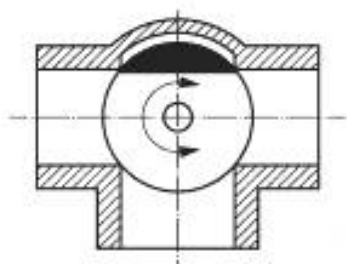
Рисунок А.5 — Горизонтальный тип, Т-образное отверстие
