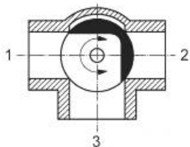
Рисунок А.10 — Ход 2 закрыт, ходы 1 и 3 соединены
