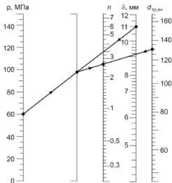
Рисунок 1 — Номограмма для определения числа ниток ДШ ТФ типа ТШ при ликвидации прихватов стальных буровых труб
