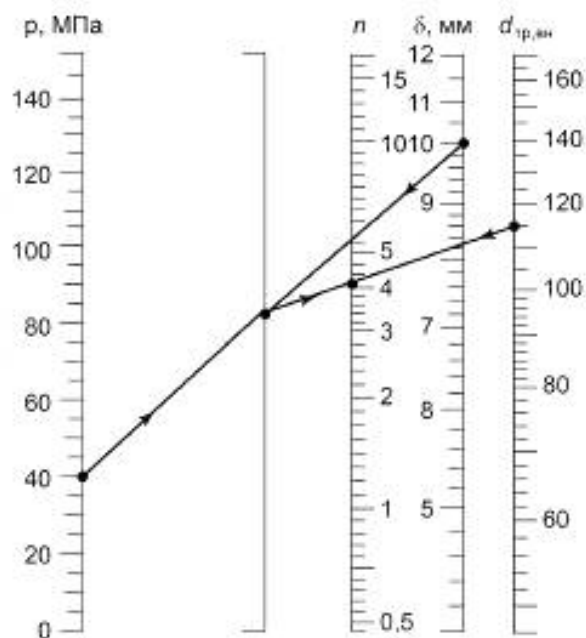
Рисунок 2 — Номограмма для определения числа ниток ДШ ФТ типа ТШ при ликвидации прихватов буровых труб из алюминиевого сплава Д16Т
