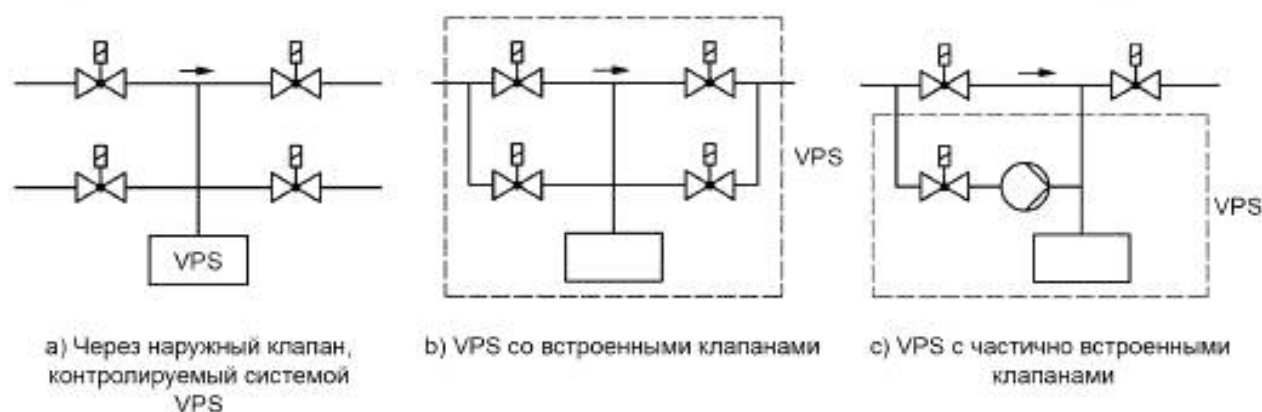
Рисунок 2 — Примеры конфигурации системы VPS
