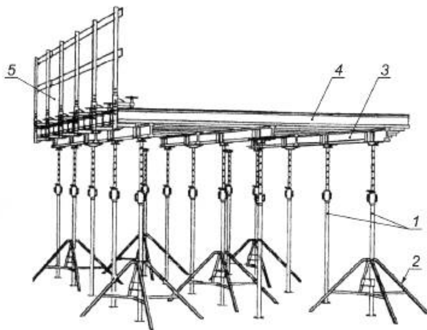
Рисунок Б.6 — Разборно-переставная опалубка перекрытий на стойках
