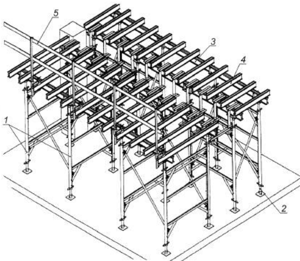
Рисунок Б.6 — Разборно-переставная опалубка перекрытий на стойках
