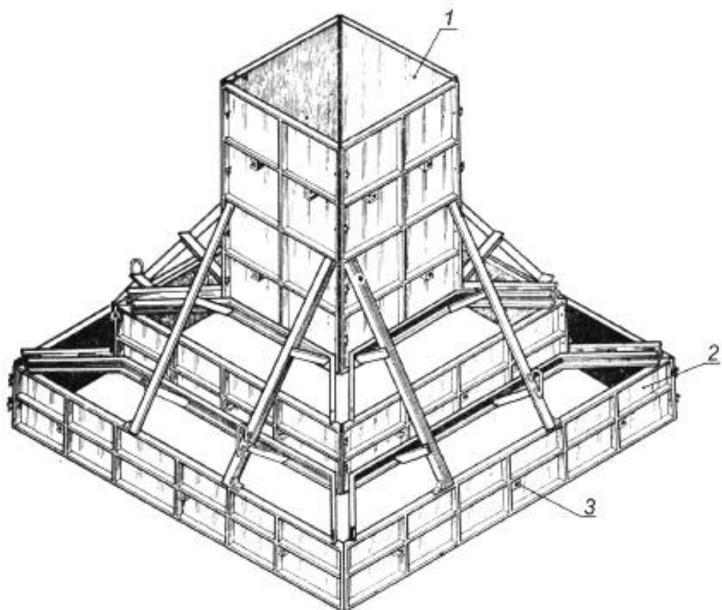
1 — опалубка подколонника; 2 — опалубка ступеней; 3 — отжимное устройство
