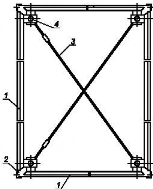
1 — щиты; 2 — угловые соединения; 3 — связи; 4 — вертикальная стойка
