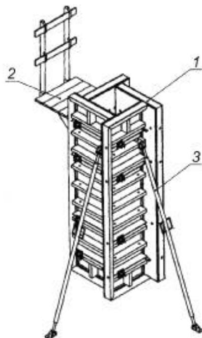
Рисунок Б.2 — Крупнощитовая модульная опалубка колонн
