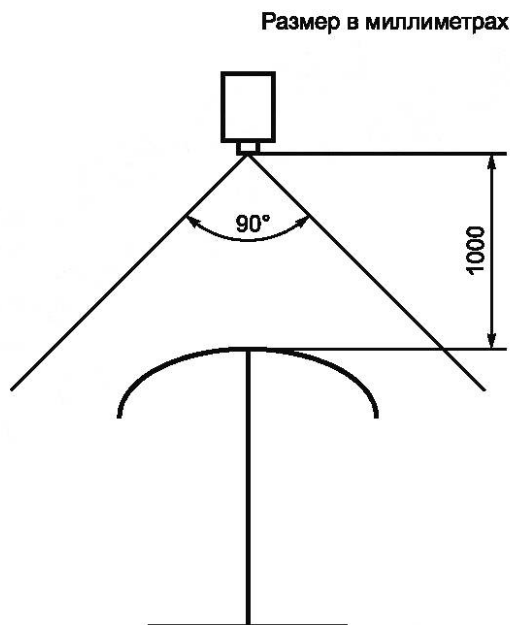
Рисунок 3 — Испытание на устойчивость к действию дождя
