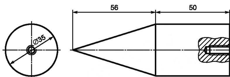
Рисунок 1 — Испытательный конус
