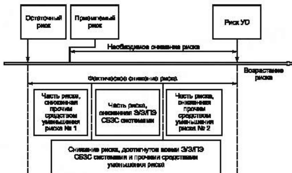
Рисунок Д.1 — Обобщенная модель снижения риска (режим с низкой частотой запросов)
