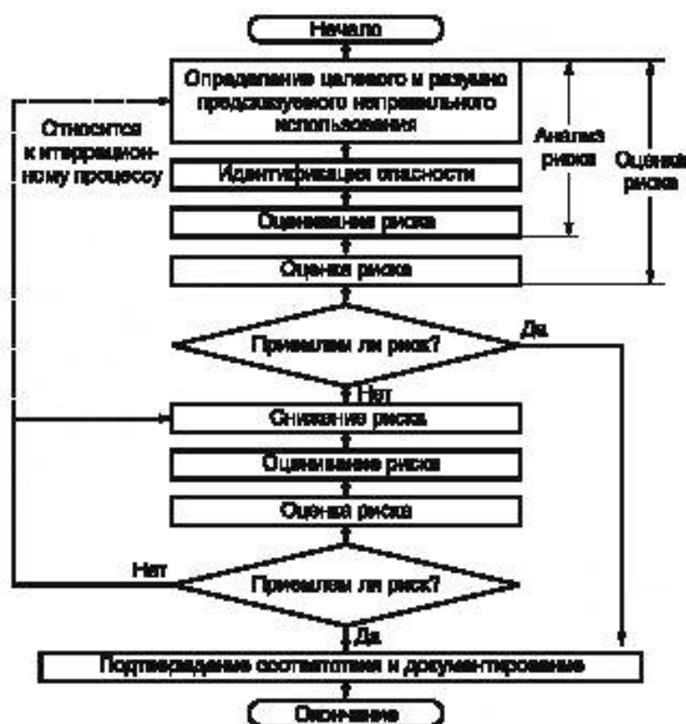
Рисунок 3 — Итерационный процесс оценки риска и снижения риска
