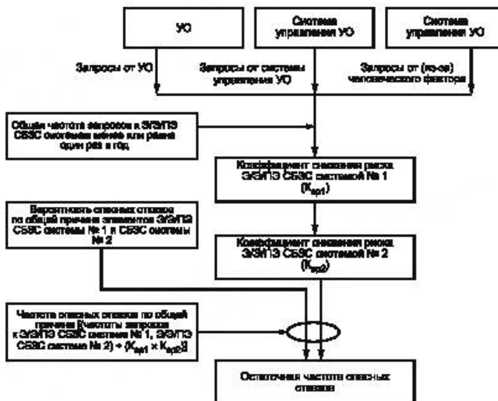
Рисунок Д.6 — Модель отказов двух Э/Э/ПЗ СБЗС систем по общей причине
