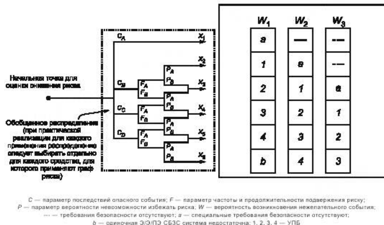
Рисунок К.1 — Общая схема графа рисков
