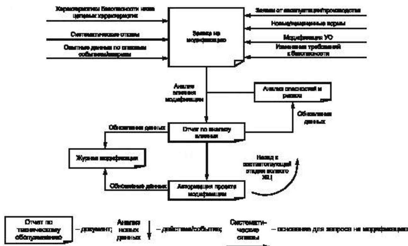
Рисунок 5 — Типичная модель процедур видоизменения (модификации) систем
