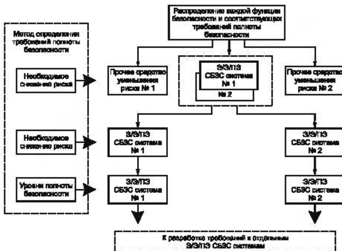
Рисунок 2 — Распределение функции безопасности по Э/Э/ПЭ СБЗС системам и другим средствам уменьшения риска
