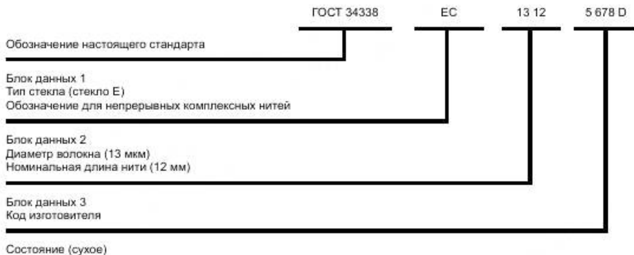
Рисунок 3 — Обозначение ГОСТ 34338-ЕС, 13 12, 5 678 D
