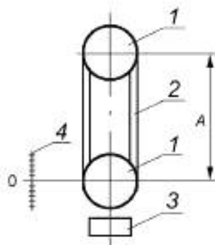
1 — верхний и нижний измерительные шкивы; 2 — клиновидный ремень; 3 — груз, обеспечивающий заданное натяжение; 4 — шкала оптического устройства для определения отклонения от номинального межцентрового расстояния
