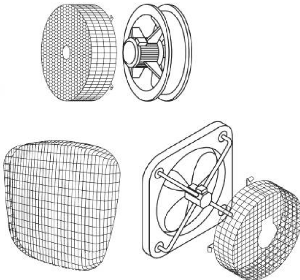
Рисунок 3 — Защитные устройства для осевого вентилятора
