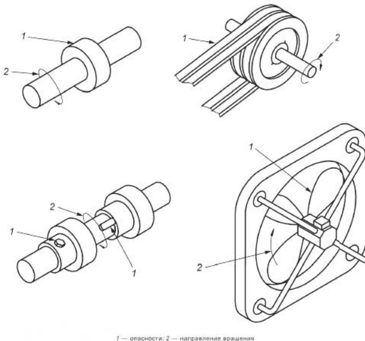
Рисунок 2 — Типичные механические опасности при эксплуатации вентиляторов [перечисления а) — д)]
